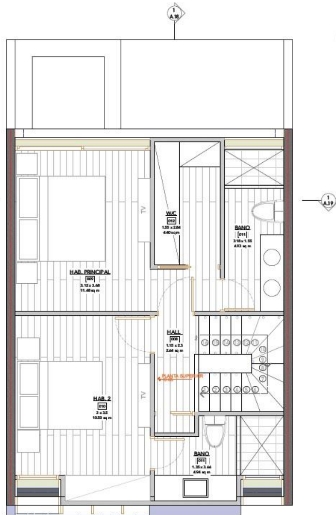
A2 Planta Arquitectonica Casa Tipo A (Planta Alta) Scale: 1:25
