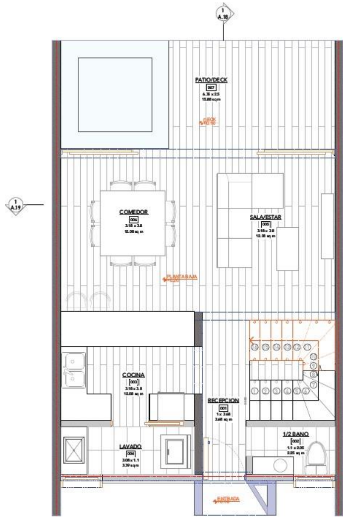
A1 Planta Arquitectonica Casa Tipo A (Planta Baja) Scale: 1:25
