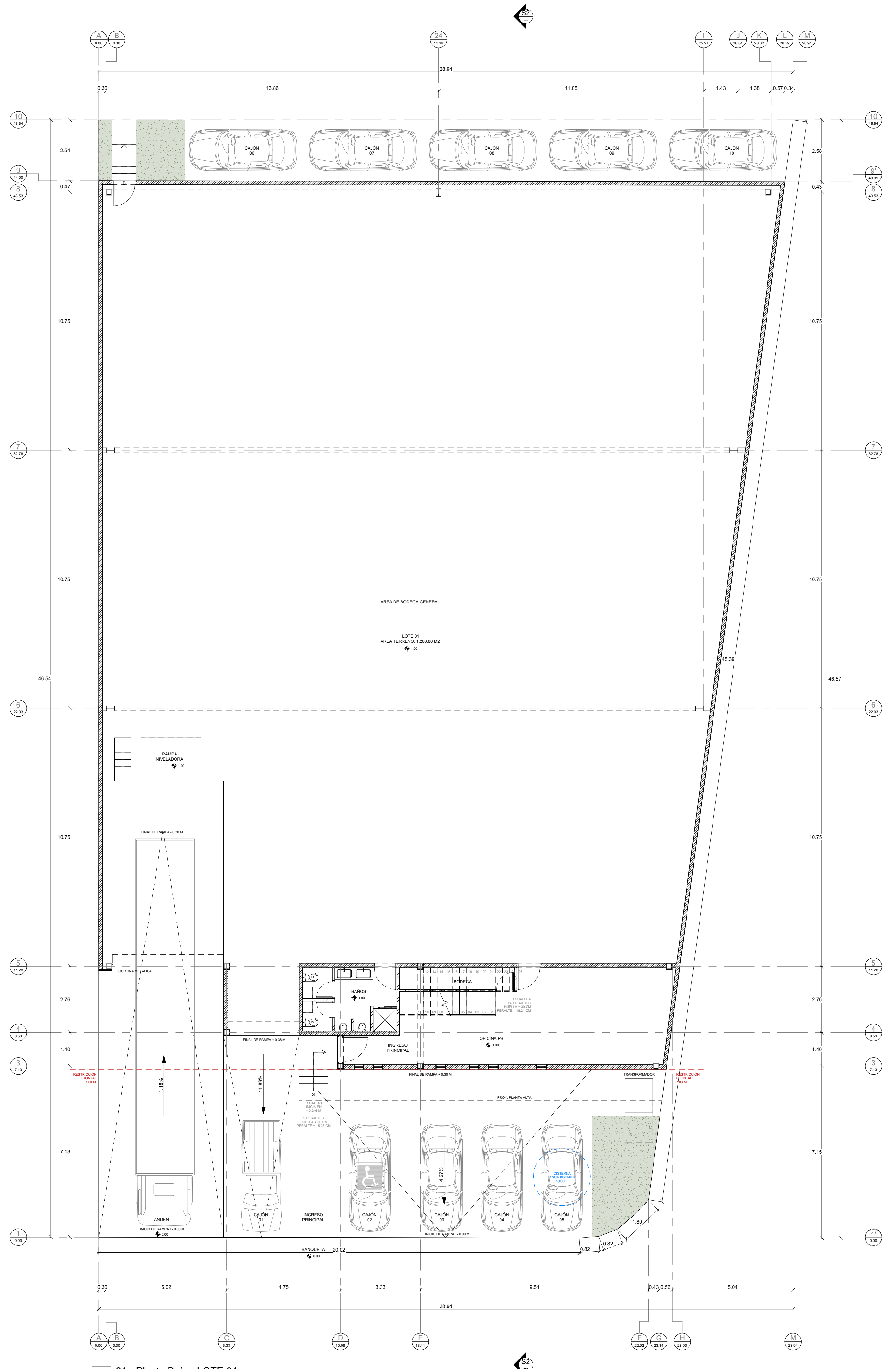
1 01 - Planta Baja - LOTE 01 1: 100
