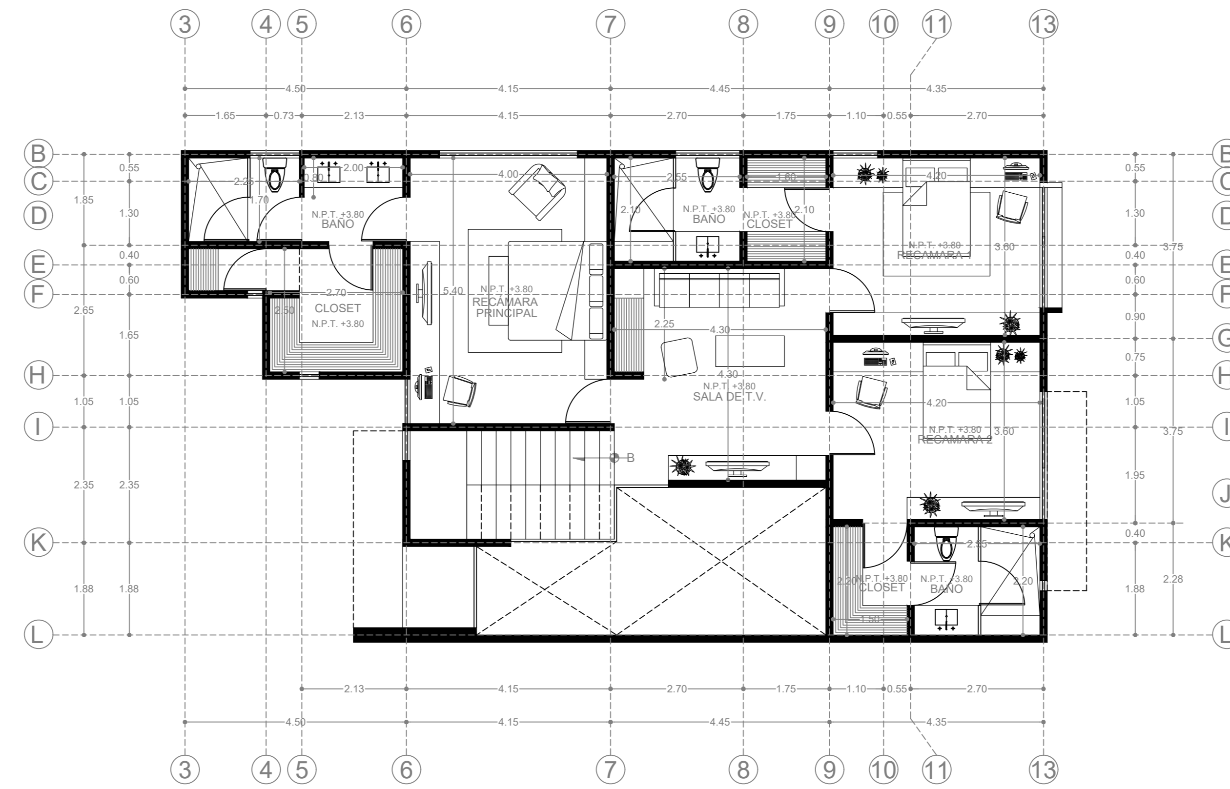
PLANTA ALTA
