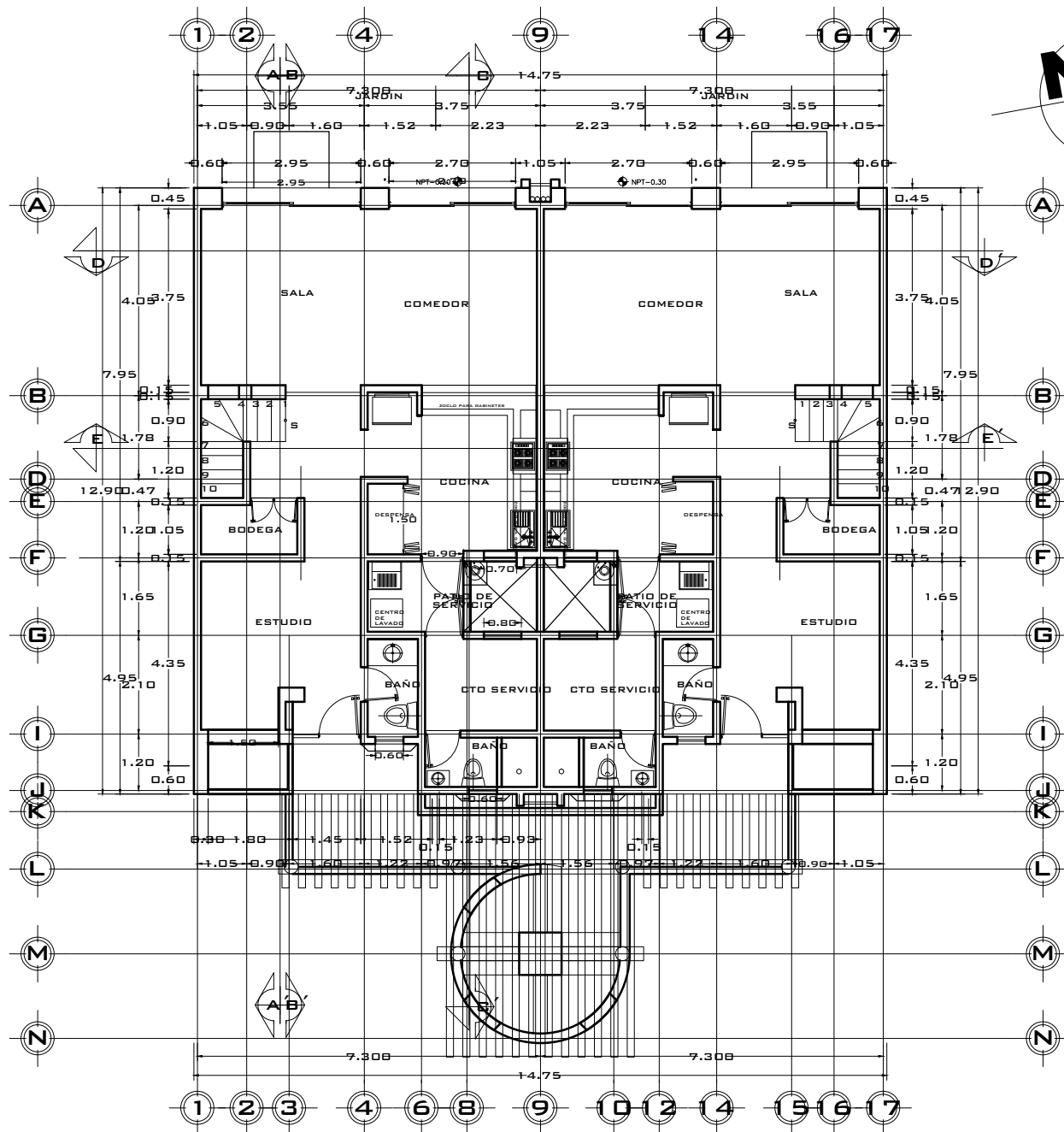
PLANTA NIVEL +5.76 VILLA TIPO
