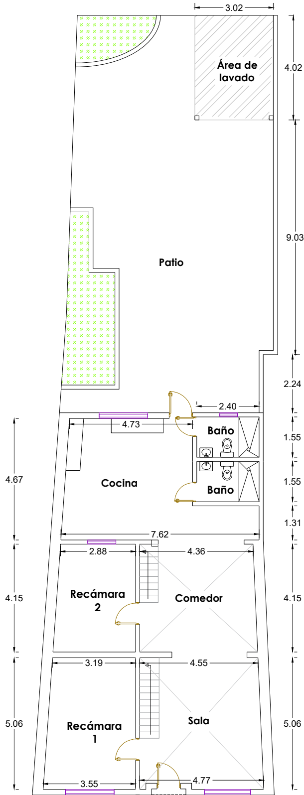
PLANTA BAJA
