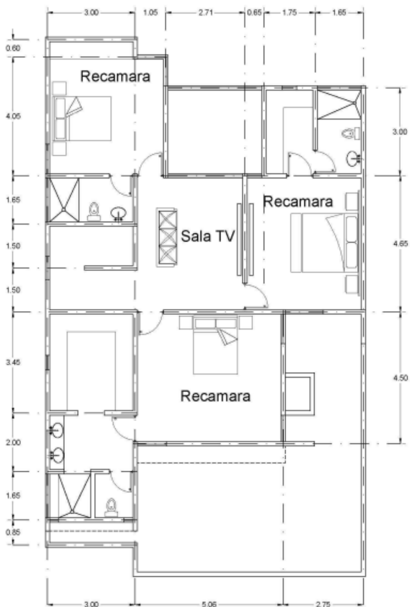
PLANTA ARQUITECTONICA P.A. Total P.A.=131.22 m 2
