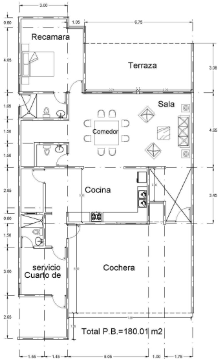
PLANTA ARQUITECTONICA P.B. Total P.B.=185.75 m2
