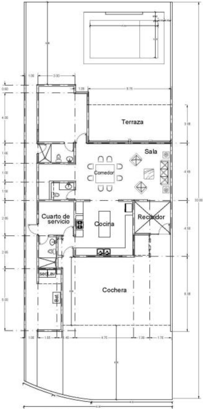
PLANTA ARQUITECTONICA P.B. 192.85 m2
