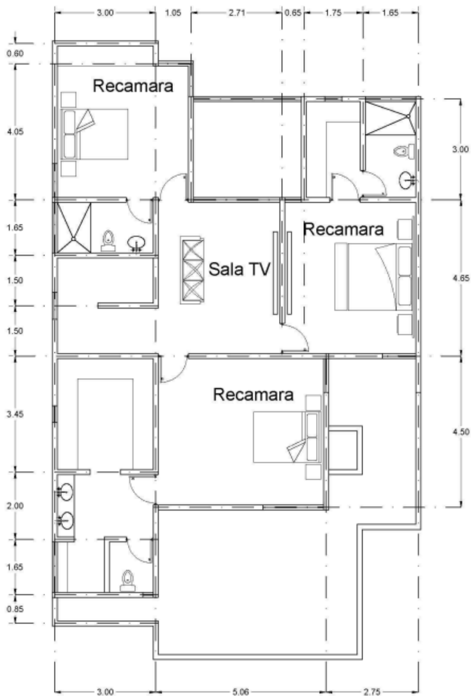
PLANTA ARQUITECTONICA P.A. Total P.A.=127.33 m2
