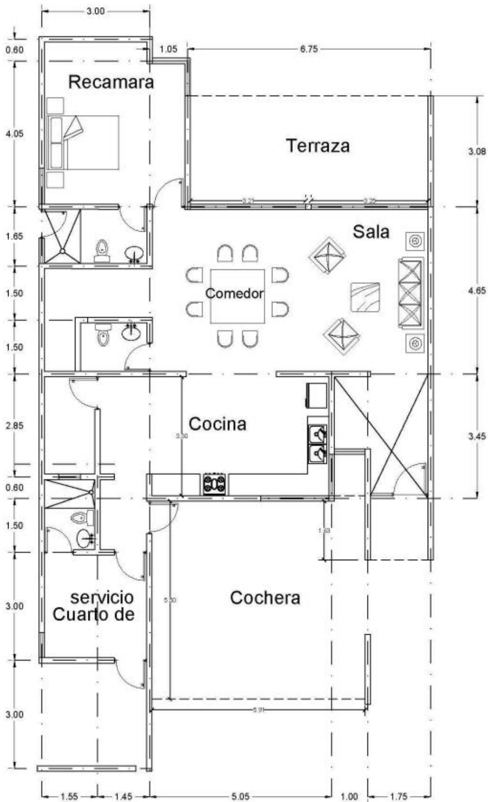
PLANTA ARQUITECTONICA P.B. Total P.B.=178.98 m2
