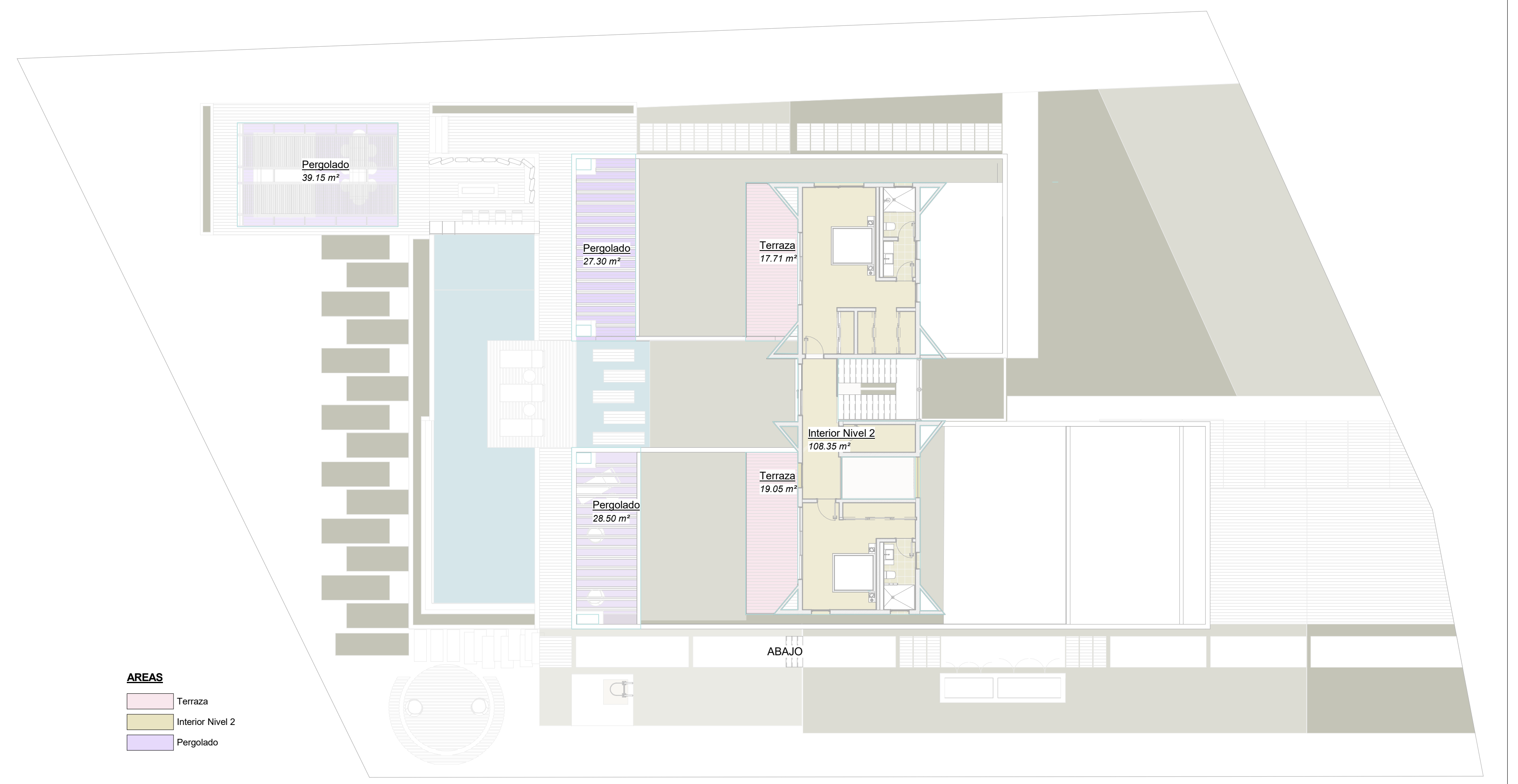
2 NIVEL 2 1 : 150
