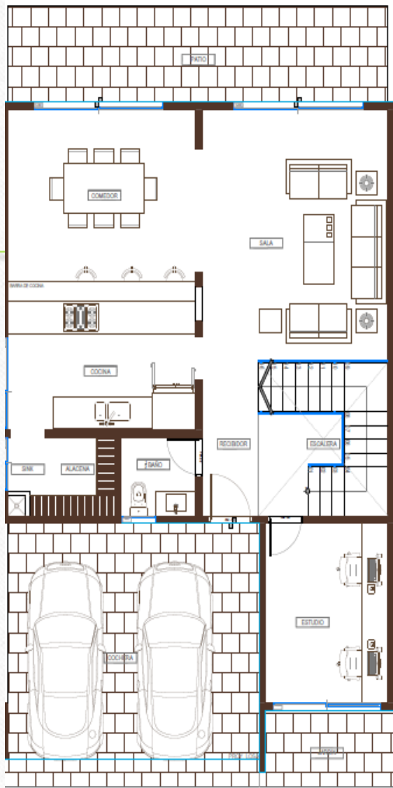
PLANTA BAJA
