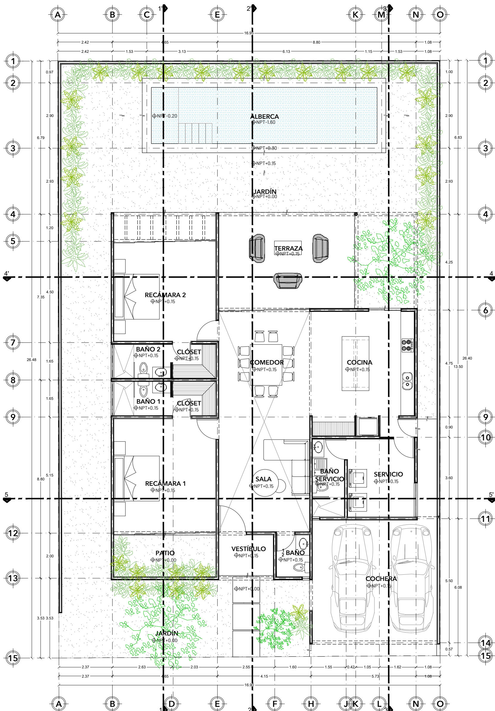
PLANTA BAJA LOTE 01 - 1:100
