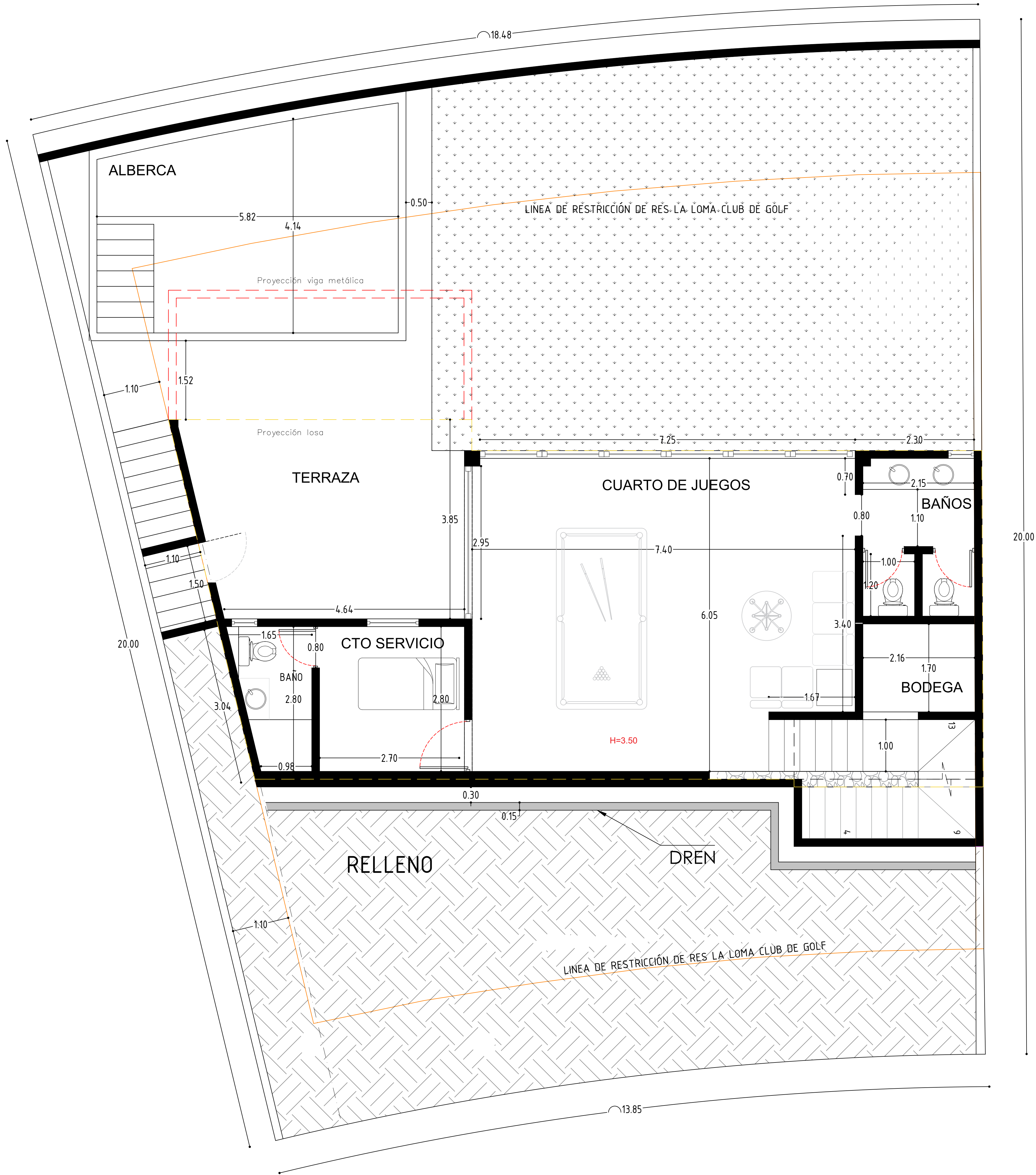
PLANTA SÓTANO
