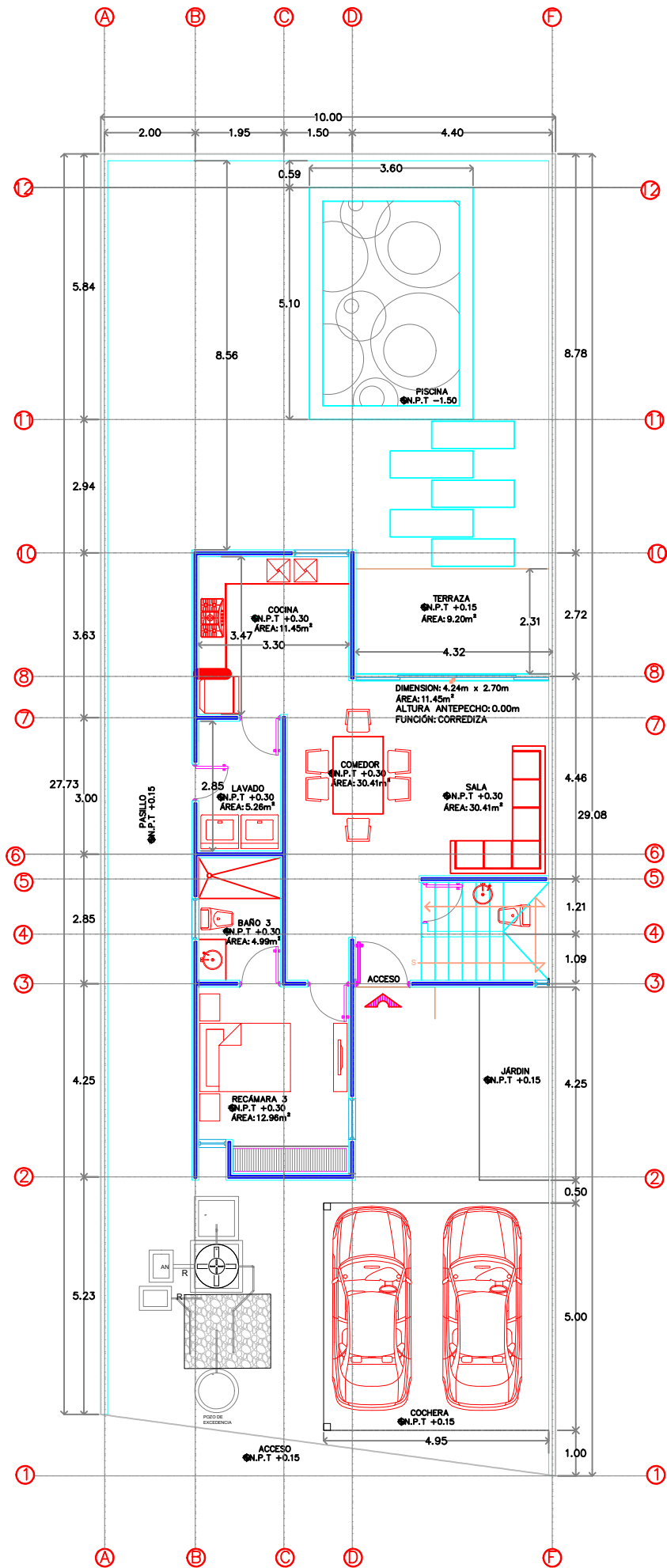
PLANTA BAJA_LOTE 72
