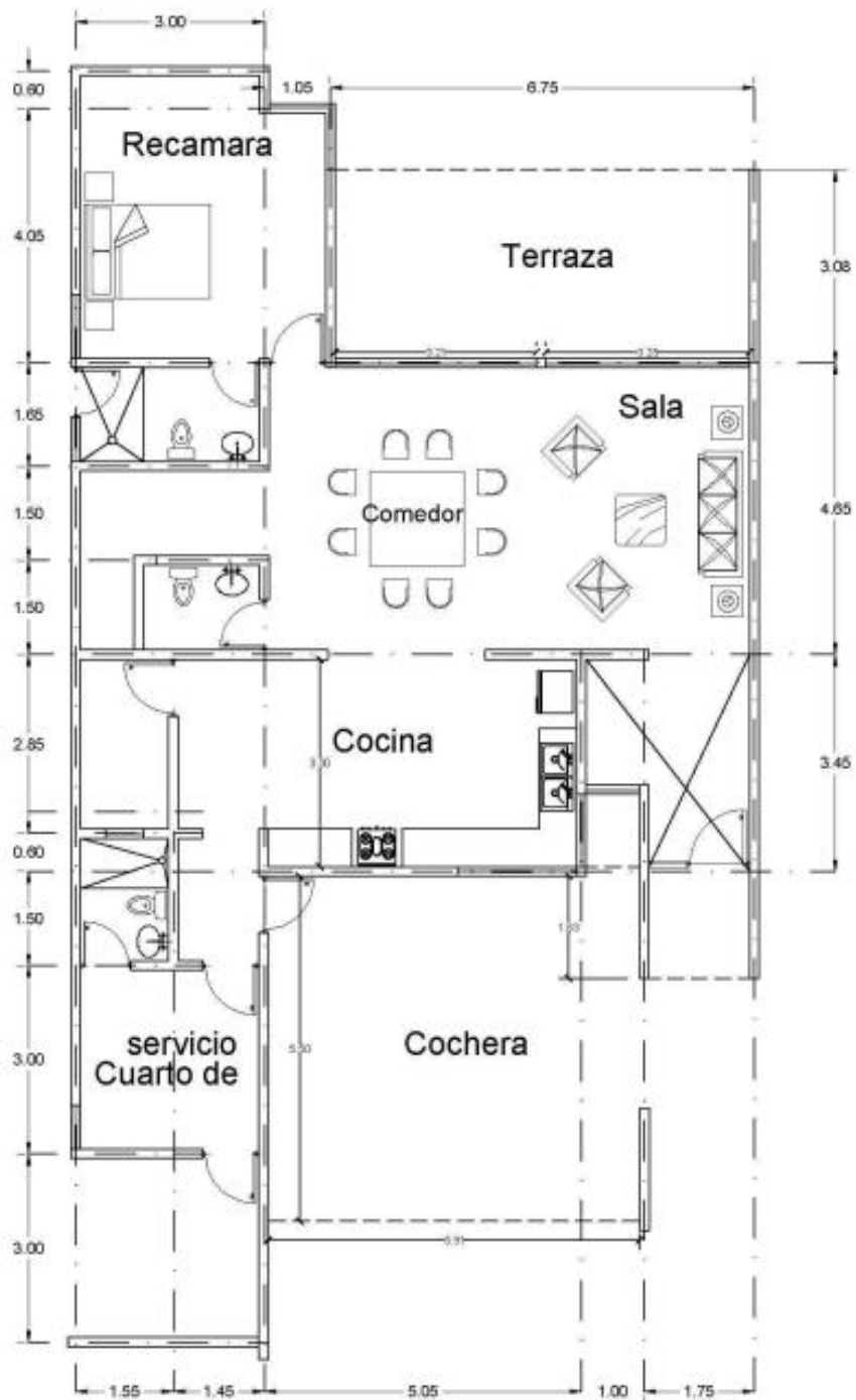
PLANTA ARQUITECTONICA P.B. Total P.B.=178.98 m 2
