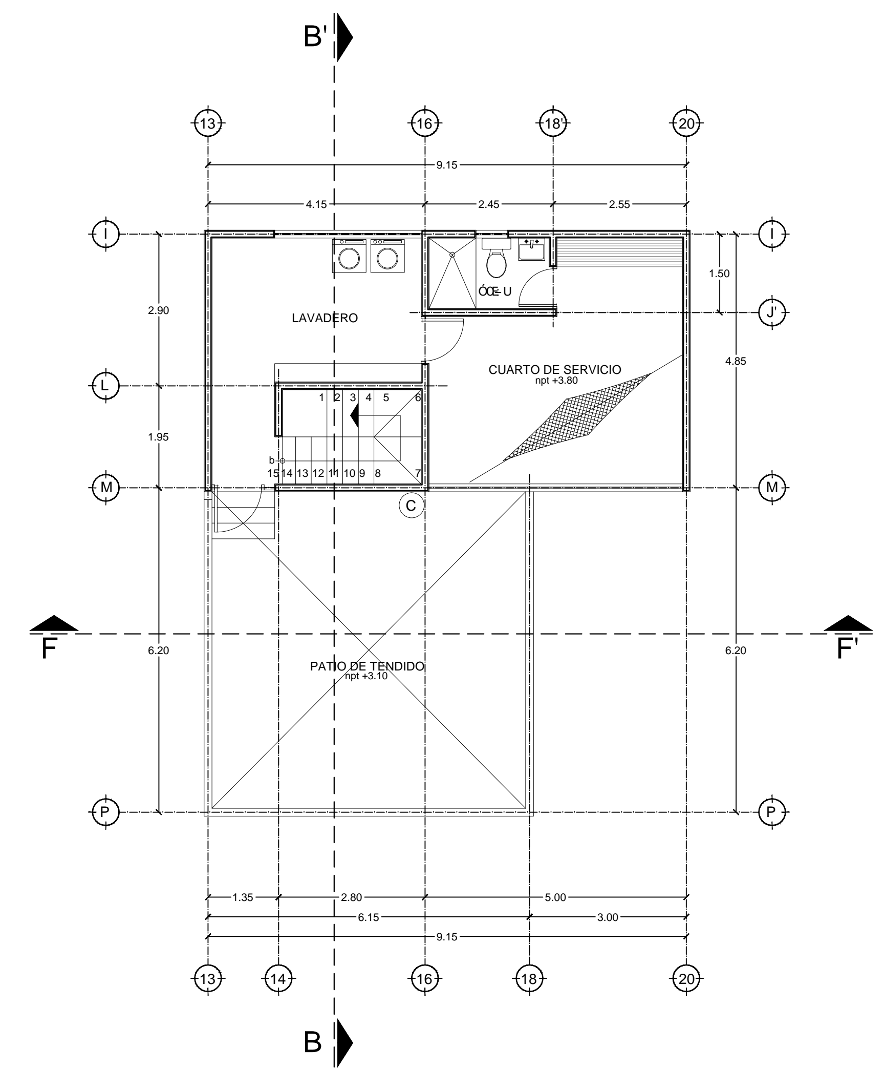
PLANTA ARQUITECTONICA ALTA
