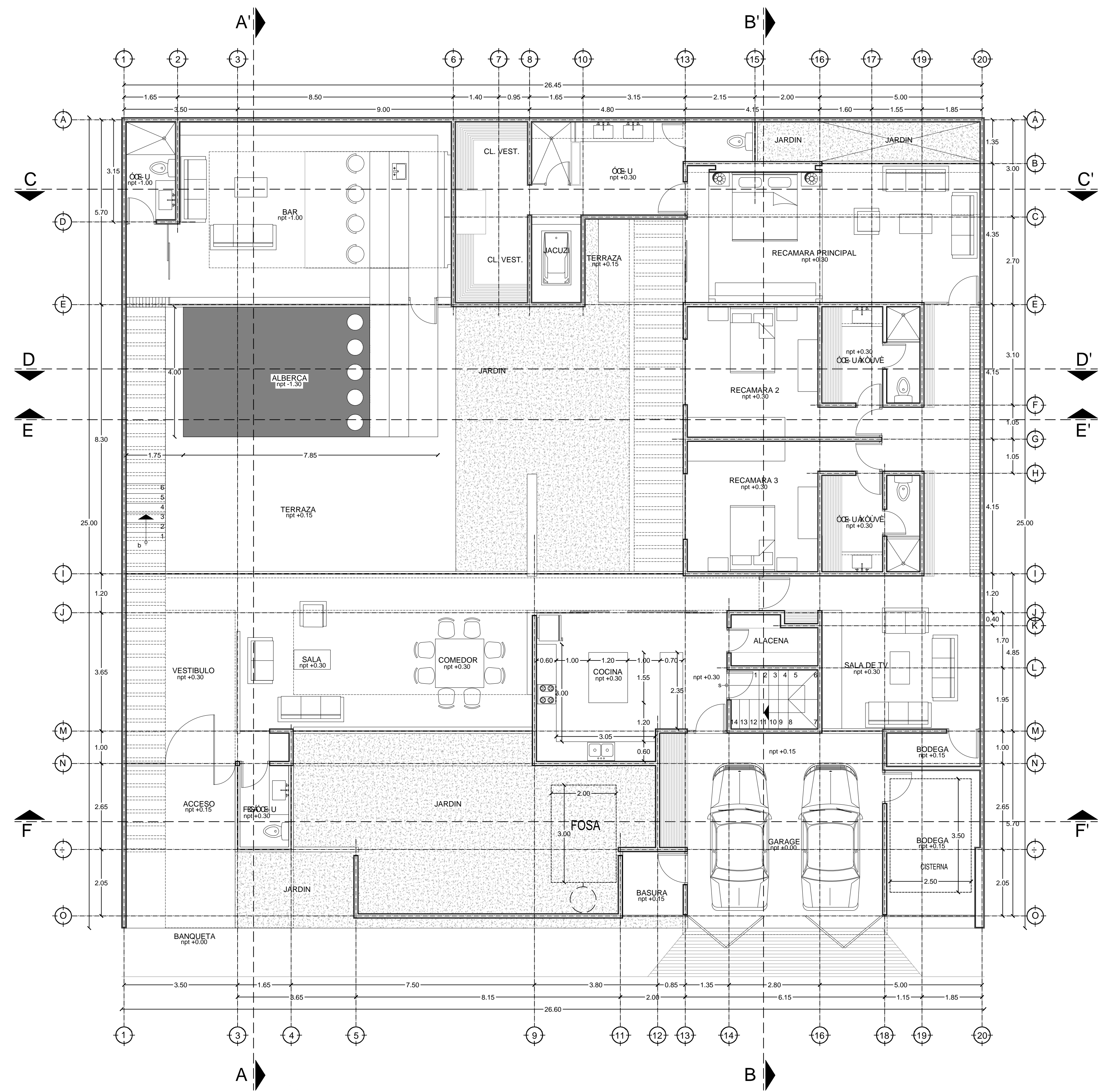
PLANTA ARQUITECTONICA BAJA
