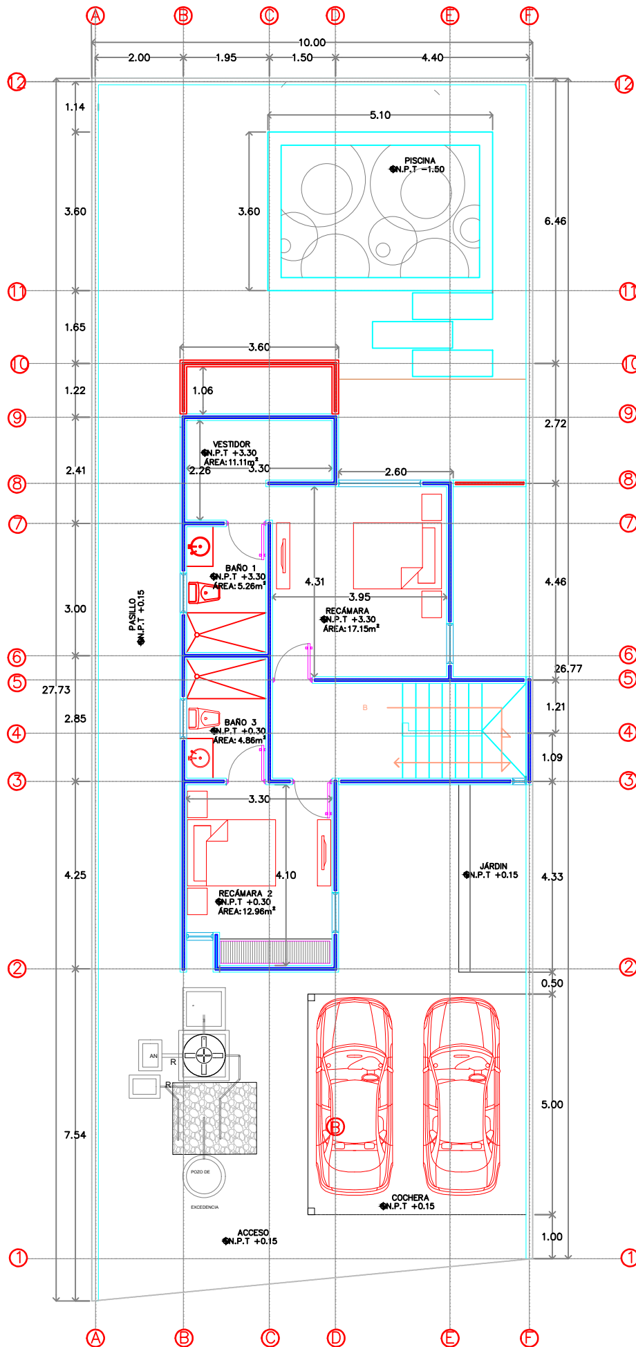
PLANTA ALTA_LOTE 78
