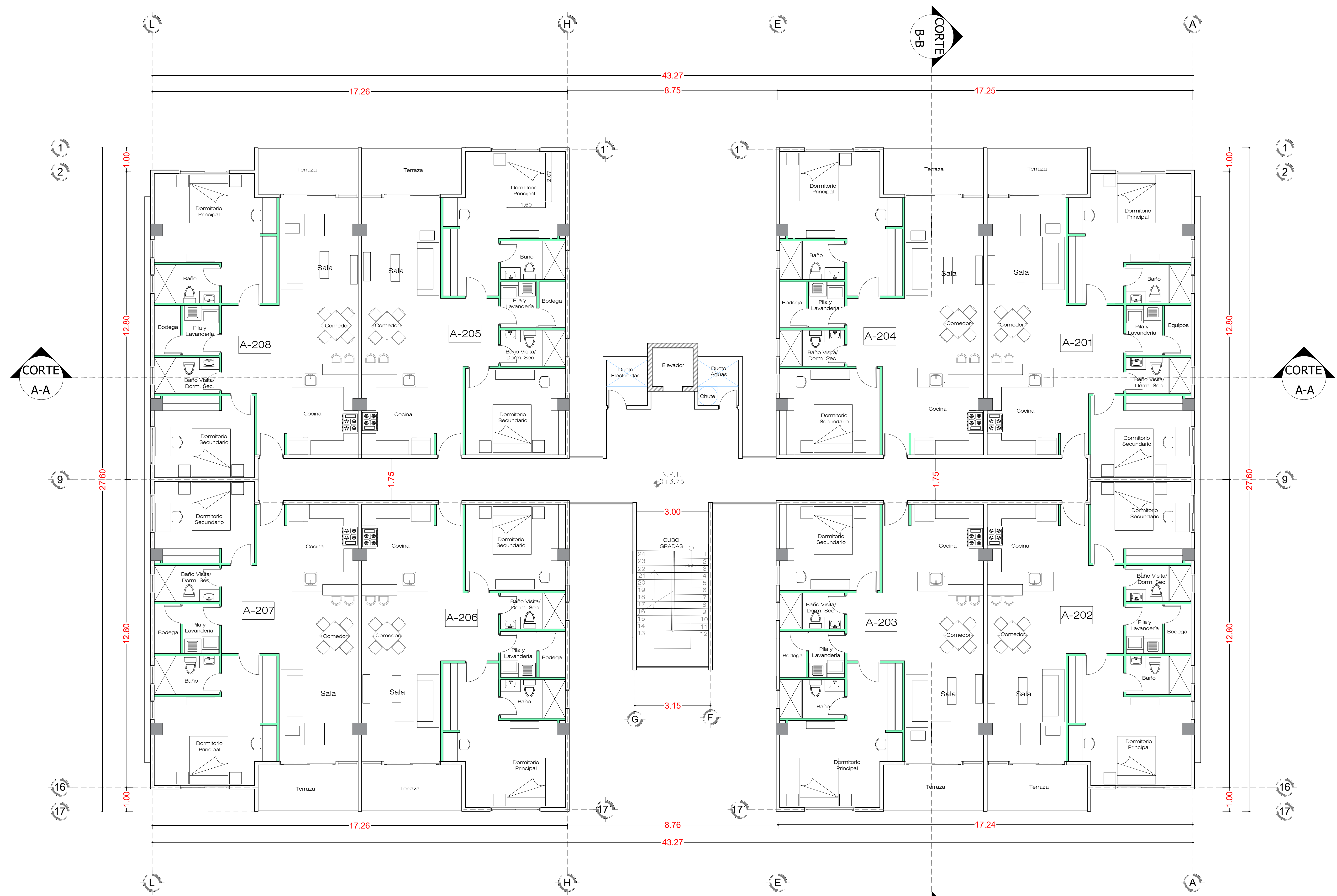
Planta Arquitectonica 2 Nivel
