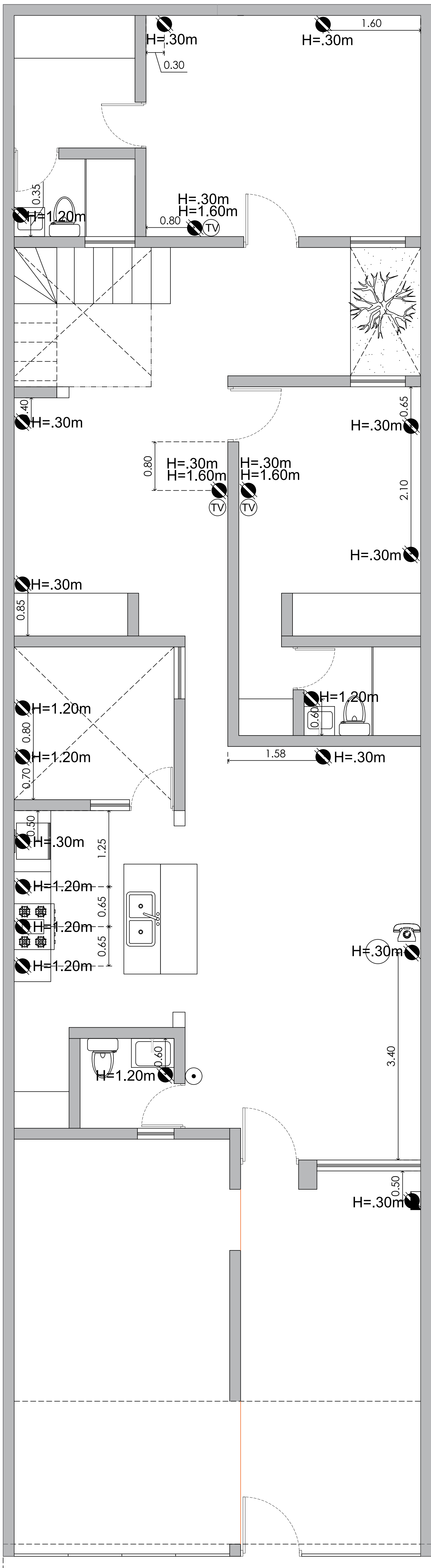
01 PLANTA ARQUITECTONICA PLANTA BAJA PROPUESTA
