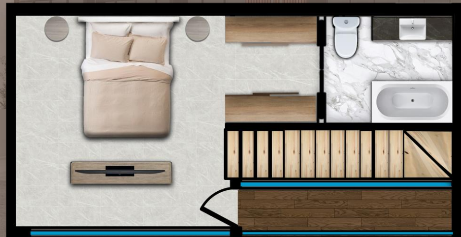
P-A. Planta alta
