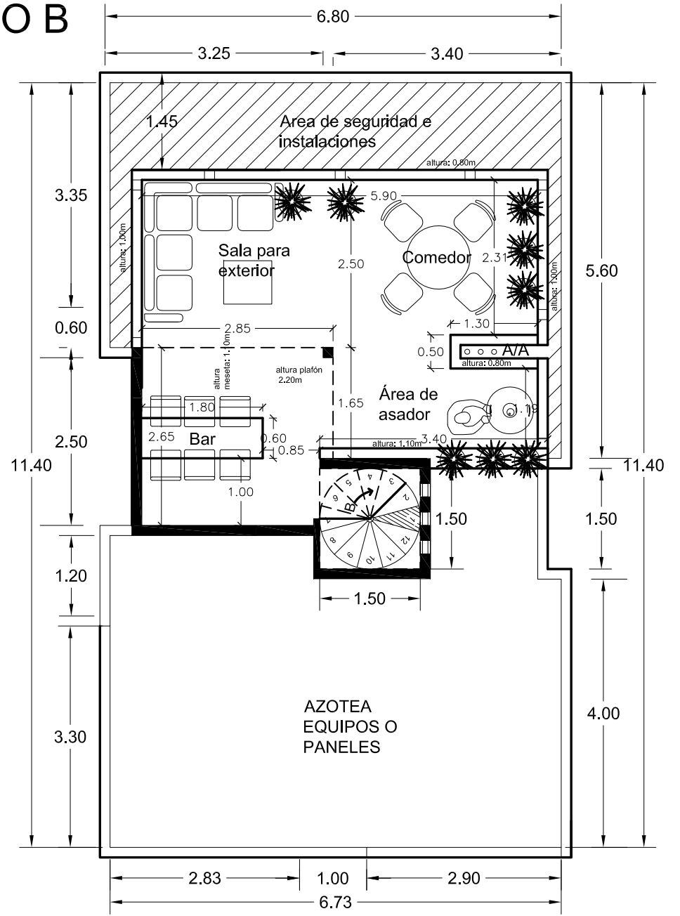
PLANTA AZOTEA
