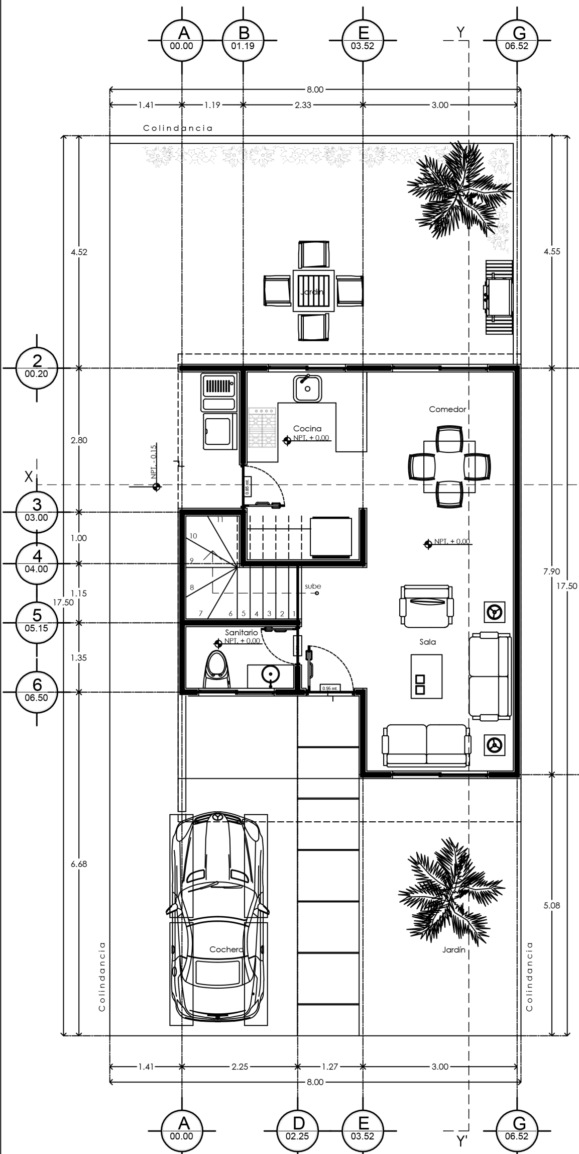
Planta Arquitectónica Baja | 48.41 m 2
