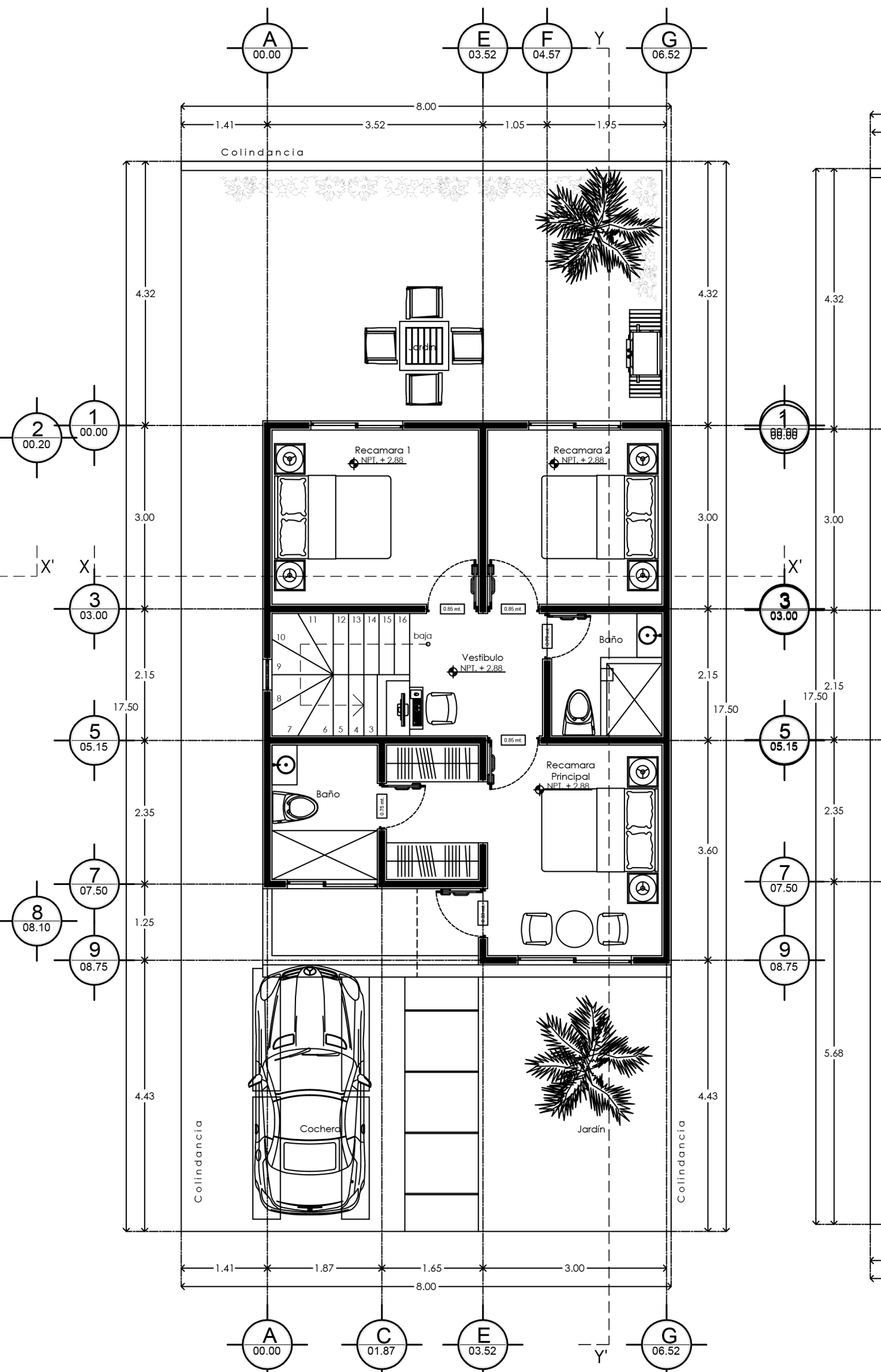
Planta Arquitectónica Alta | 54.94 m 2
