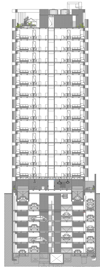
CORTE TRANSVERSAL T01
