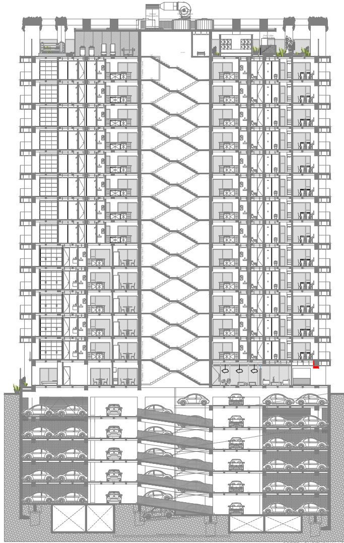
CORTE LONGITUDINAL L02
