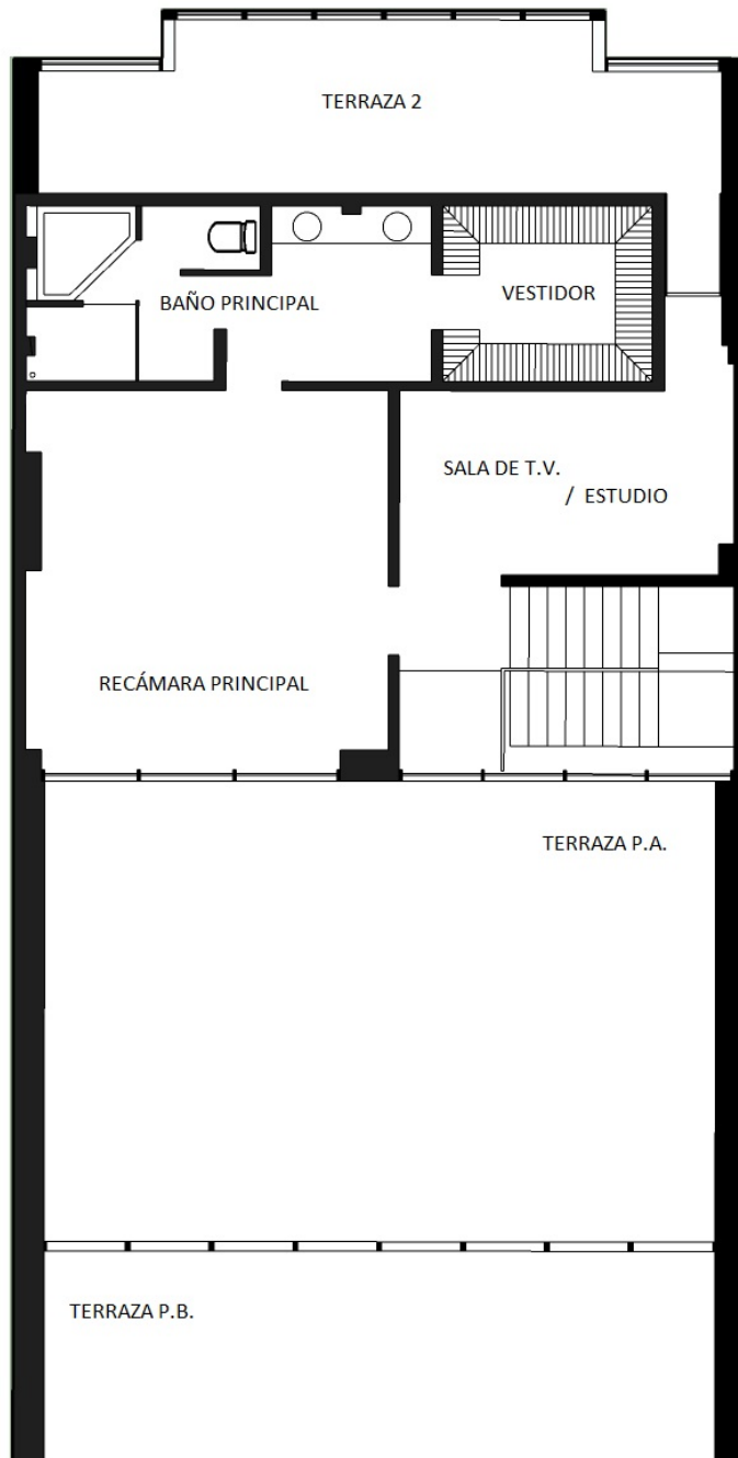
Planta Alta
