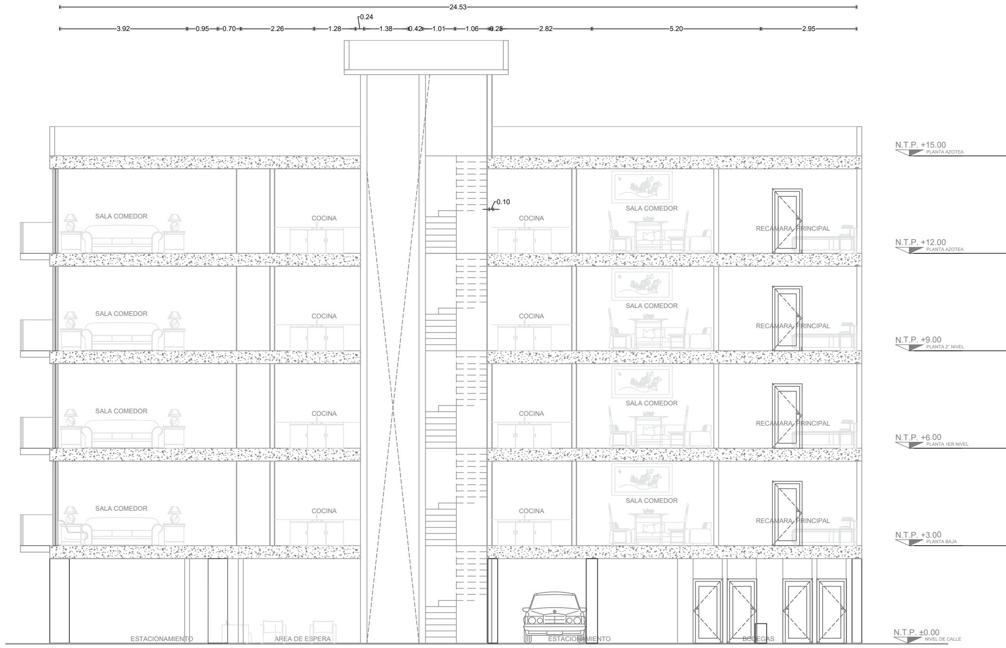
CORTE TRANSVERSAL
