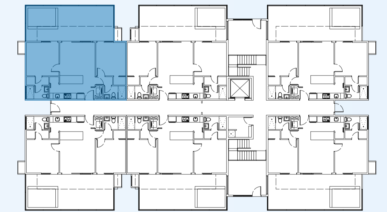
Detalle de Planta Tipo
