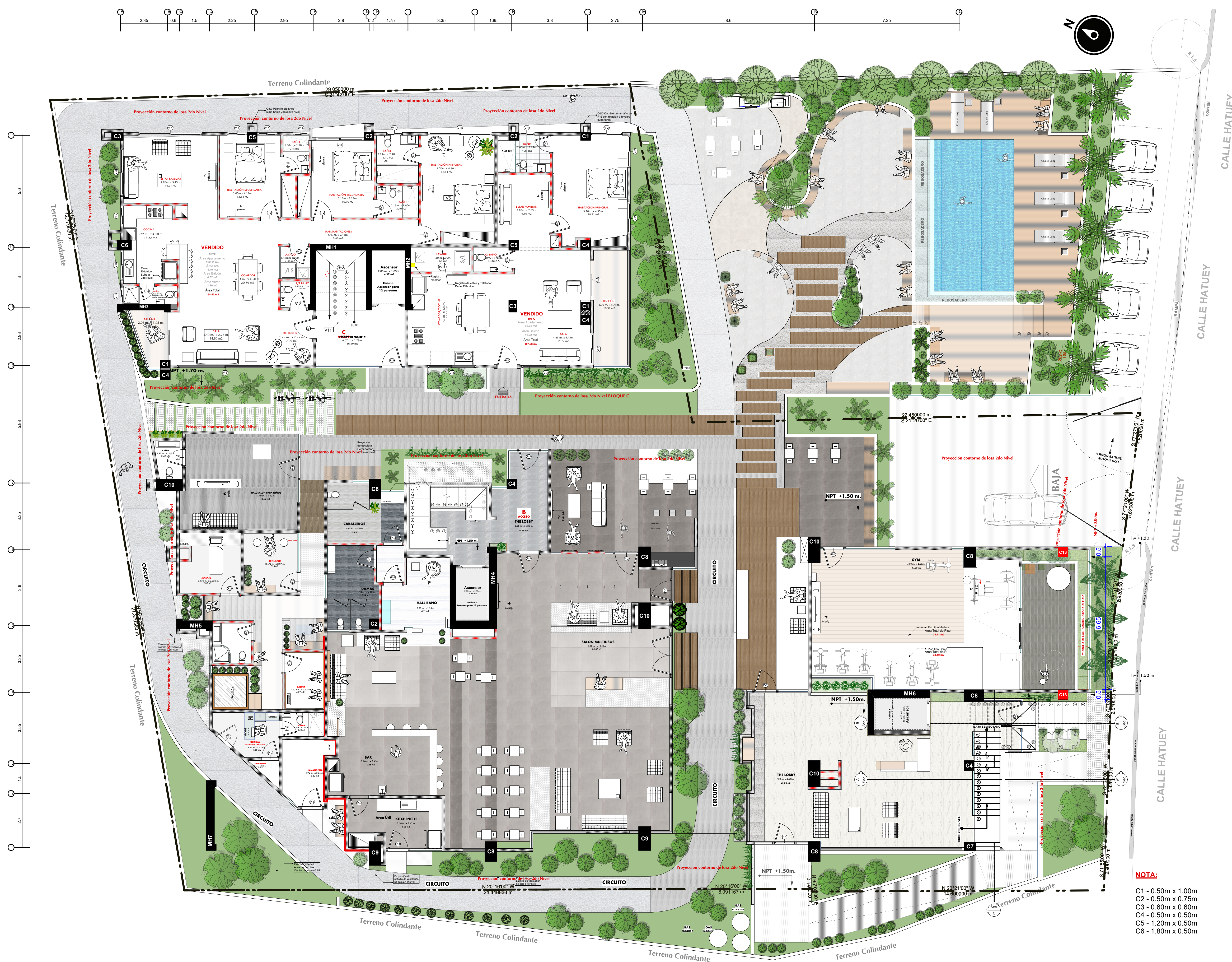
4 PLANTA ARQ. 1ER NIVEL BLOQUE ABC 14 SCALE 1:100
