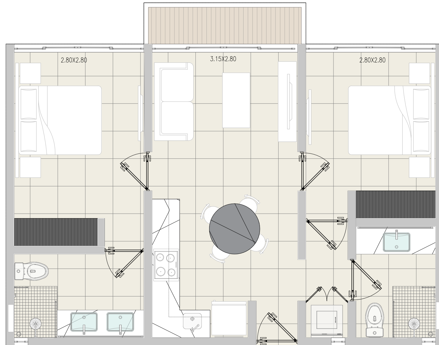
DEPARTAMENTO DOBLE 1 PA Esc: 1:50 AREA 65.90 M2
