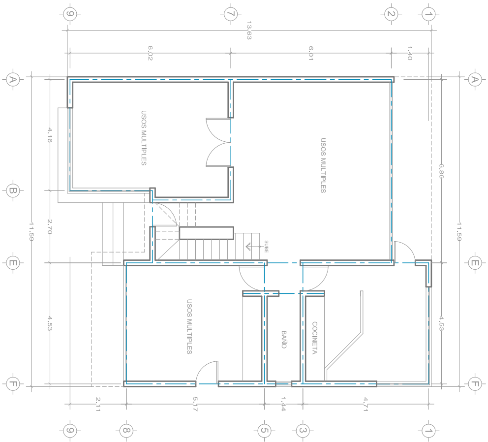
PLANTA ARQUITECTONICA BAJA EDIFICIO PRINCIPAL
