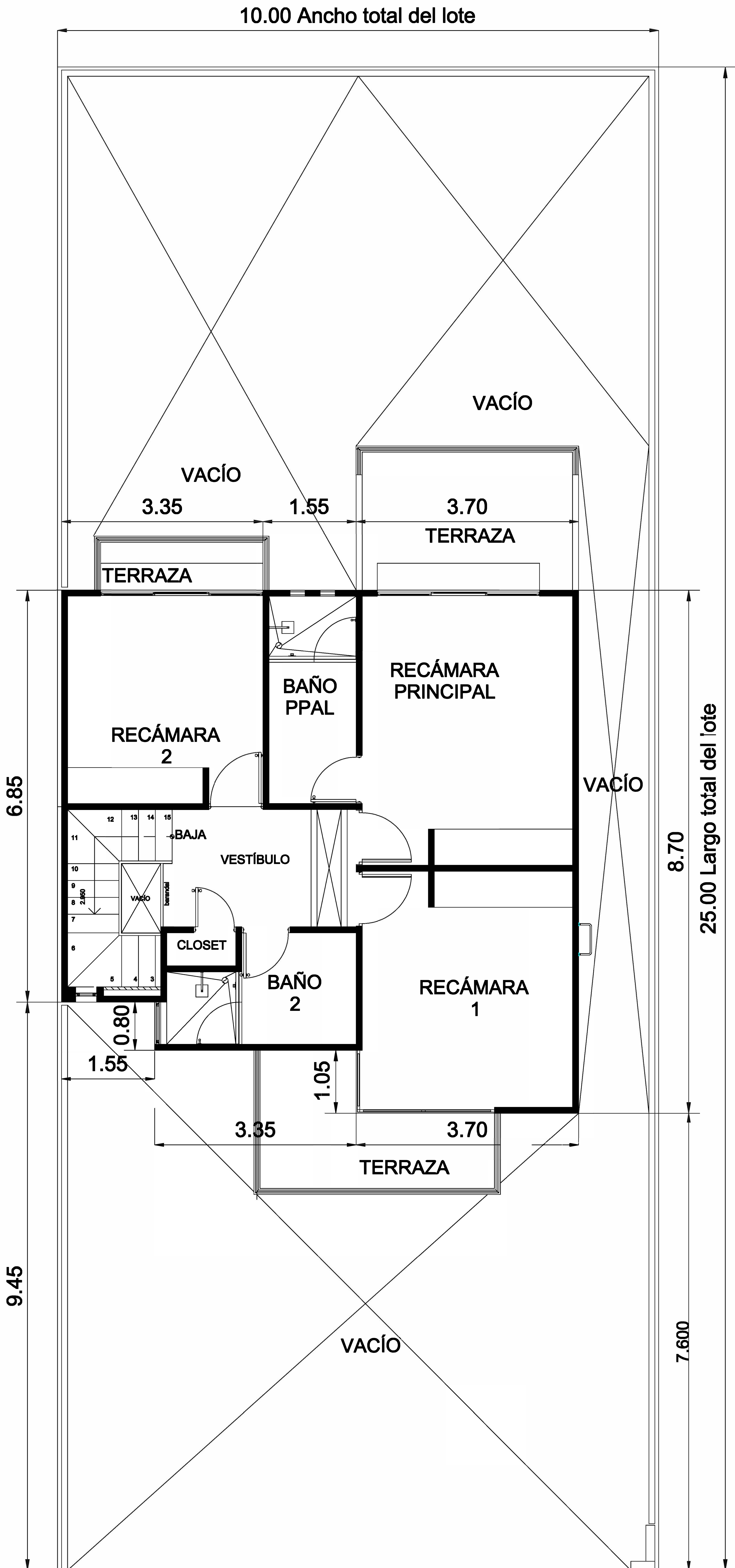
PLANTA ALTA
