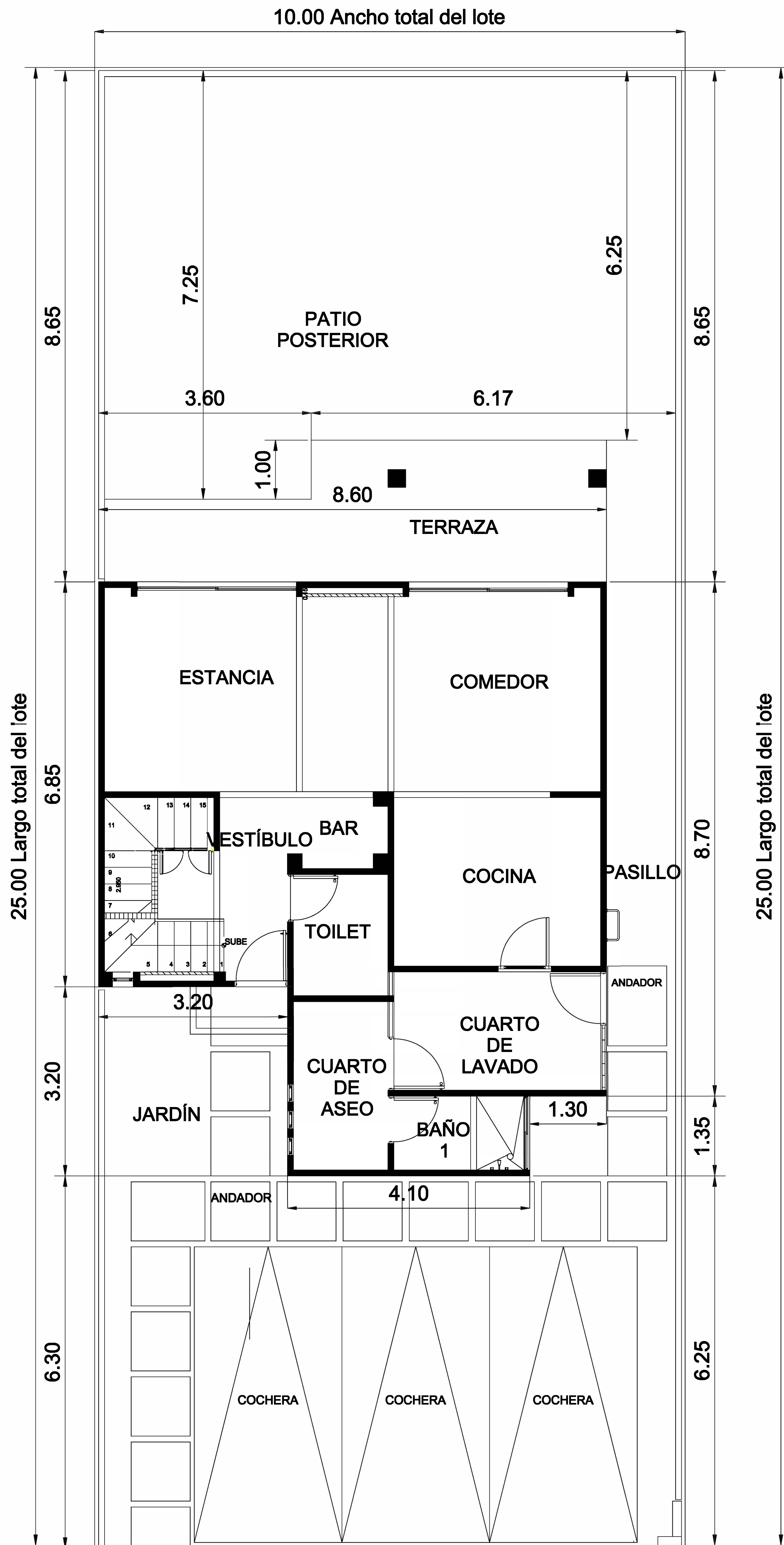
PLANTA BAJA
