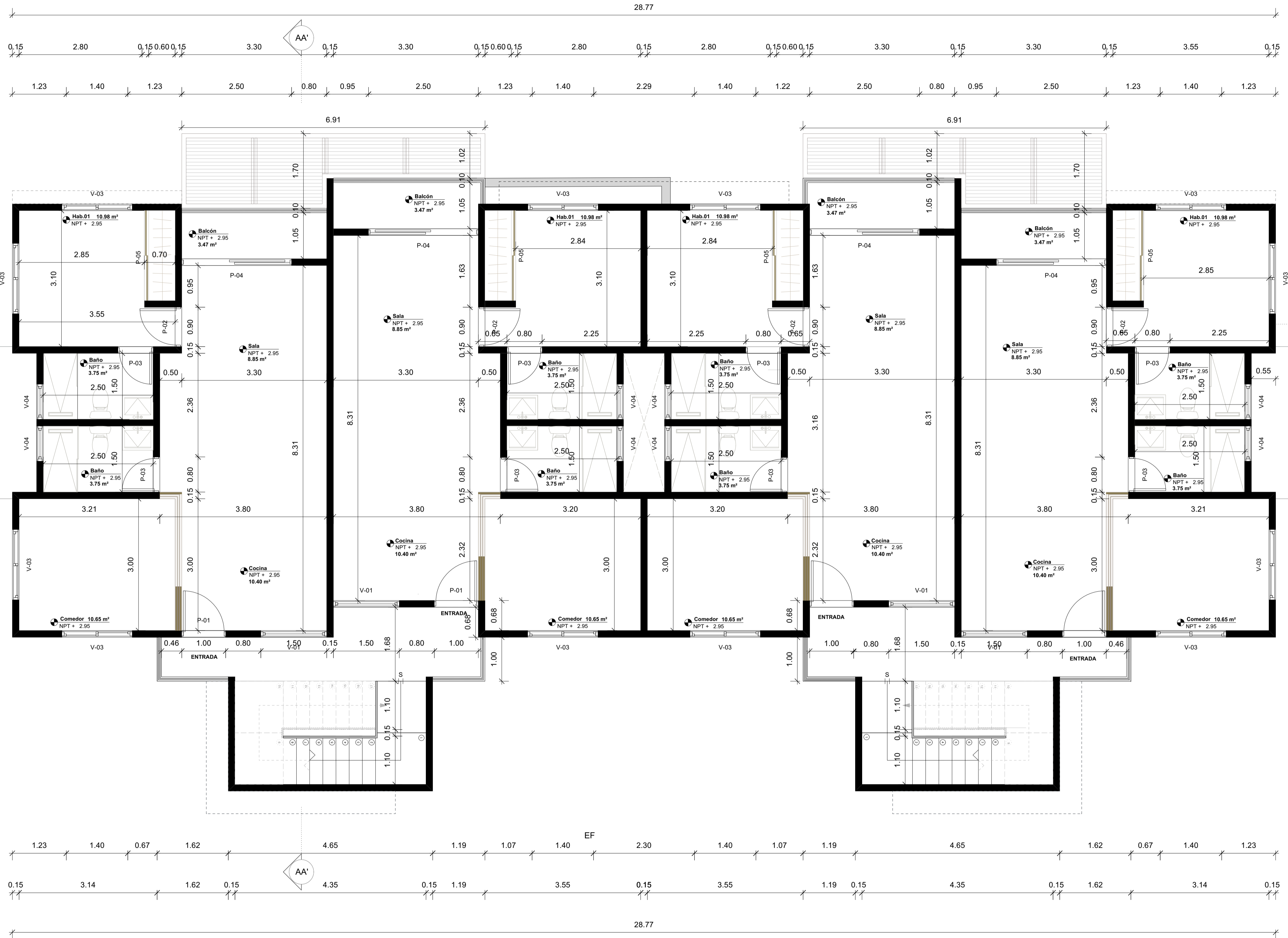
1 PLANTA DIMENSIONADA-2DO NIVEL - GAYA RESIDENCES Scale: 1:50
