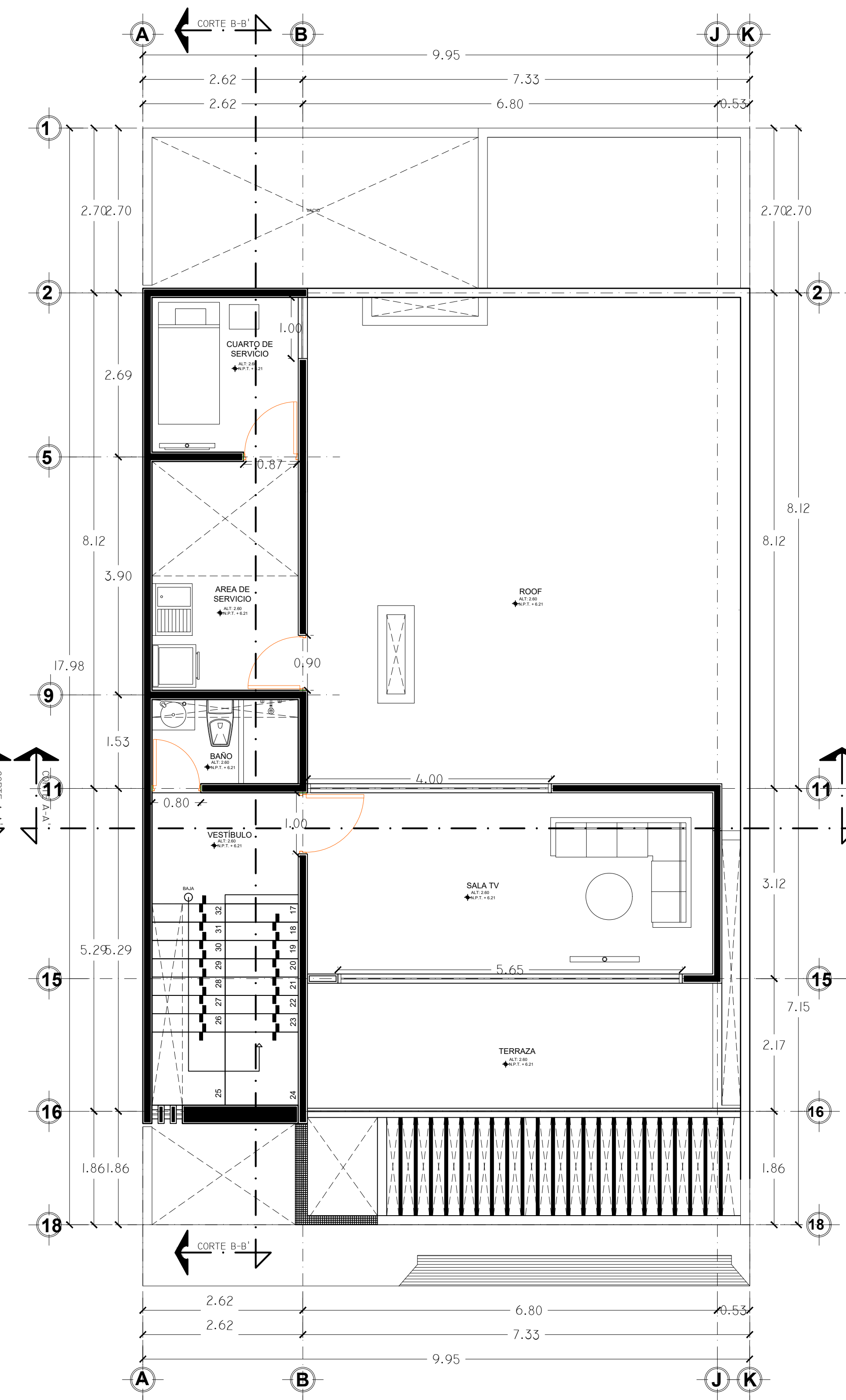
PLANTA ROOF
