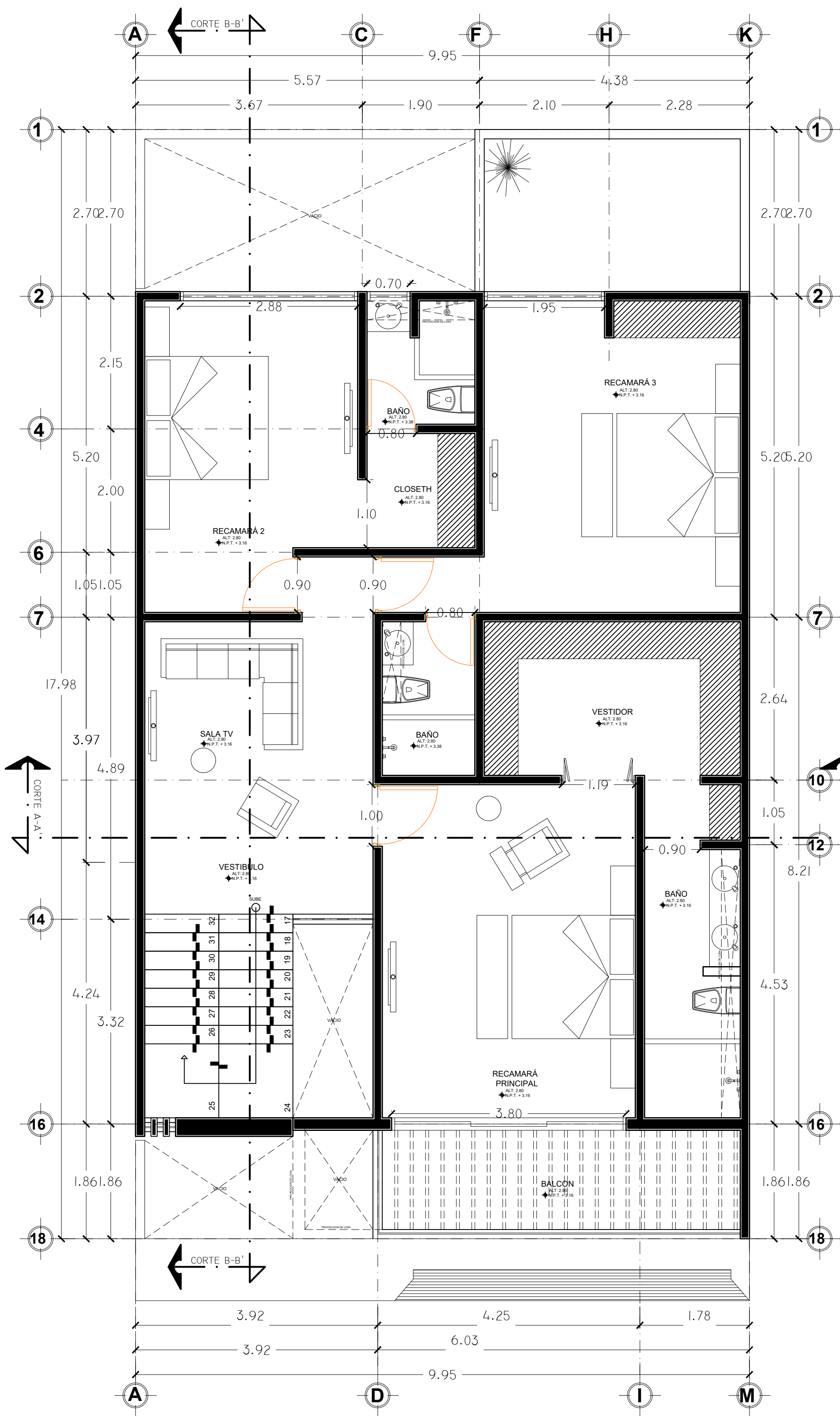
PLANTA ALTA
