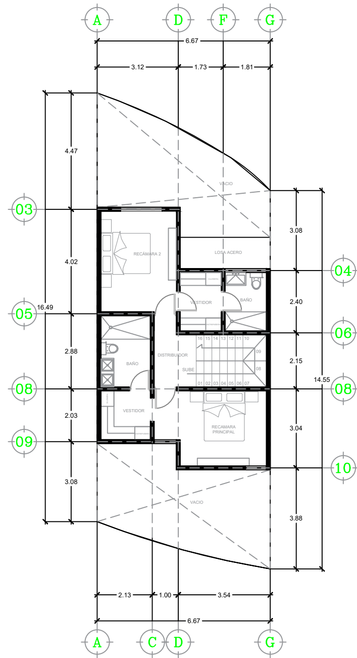
NIVEL 1
