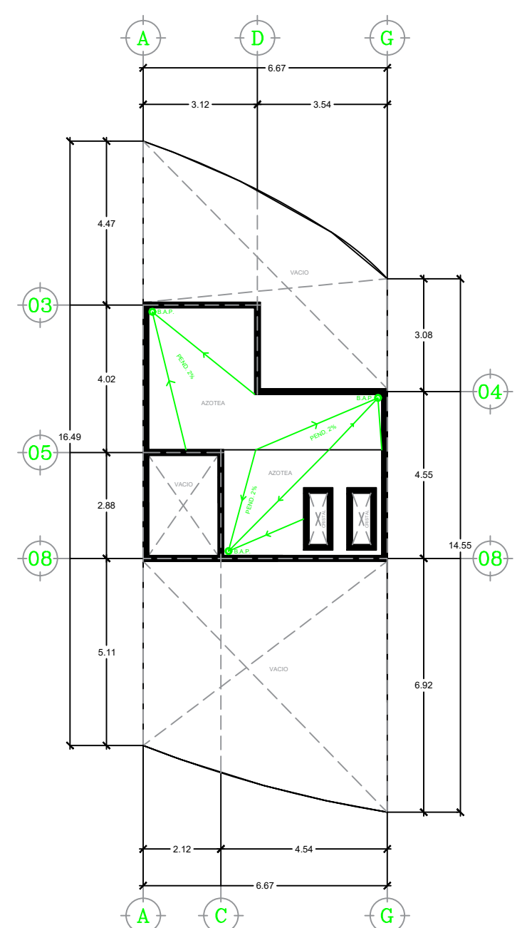
AZOTEA
