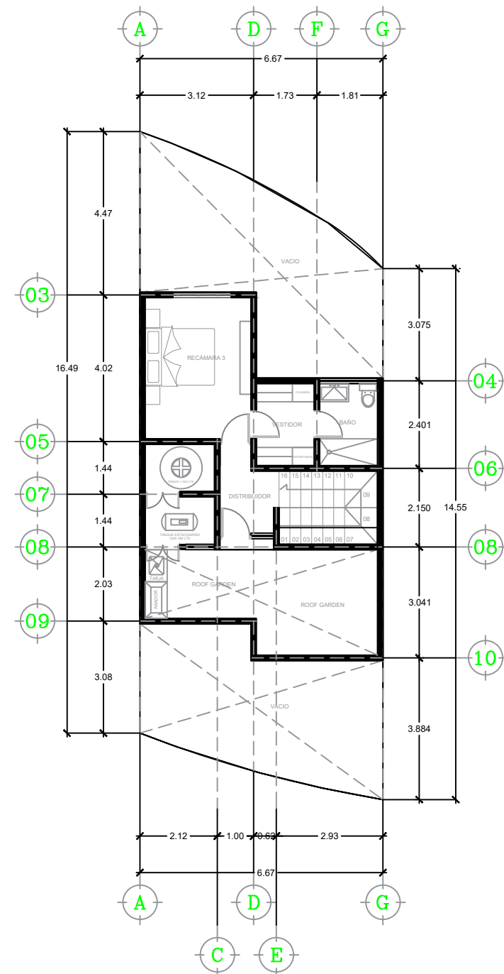
NIVEL 2
