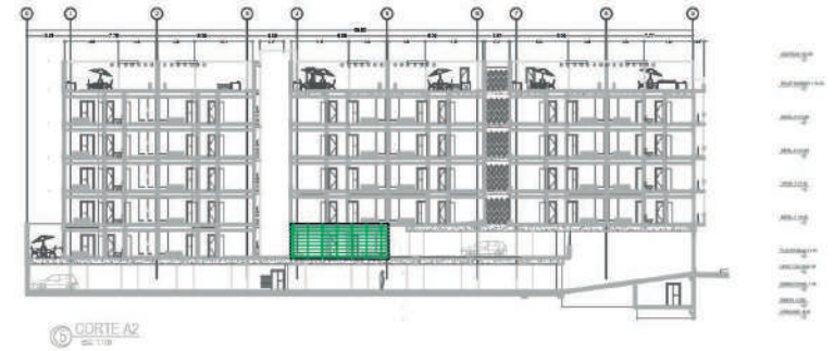
UBICACION DE DEPARTAMENTO EN CORTE ARQUITECTONICO
