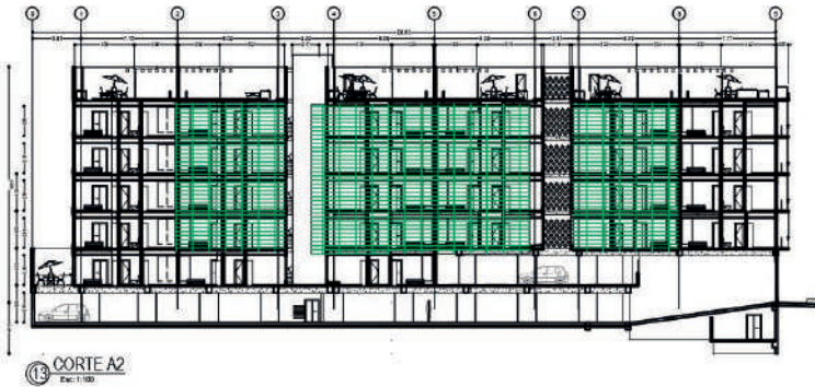
UBICACION DE DEPARTAMENTO EN CORTE ARQUITECTONICO
