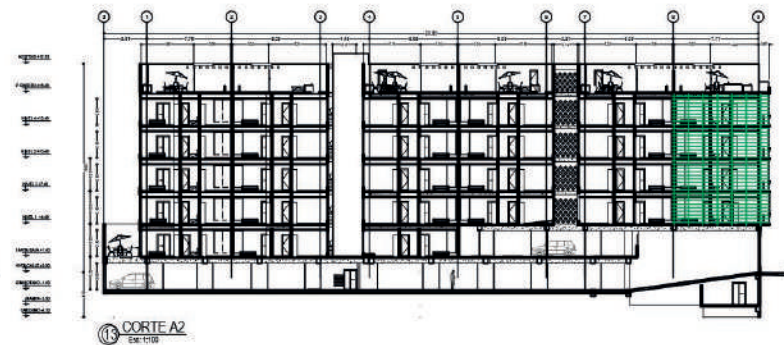
UBICACION DE DEPARTAMENTO EN CORTE ARQUITECTONICO
