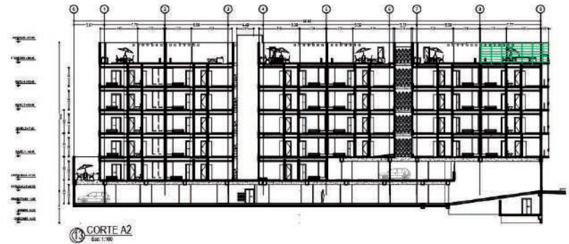
UBICACION DE ROOF GARDEN EN CORTE ARQUITECTONICO
