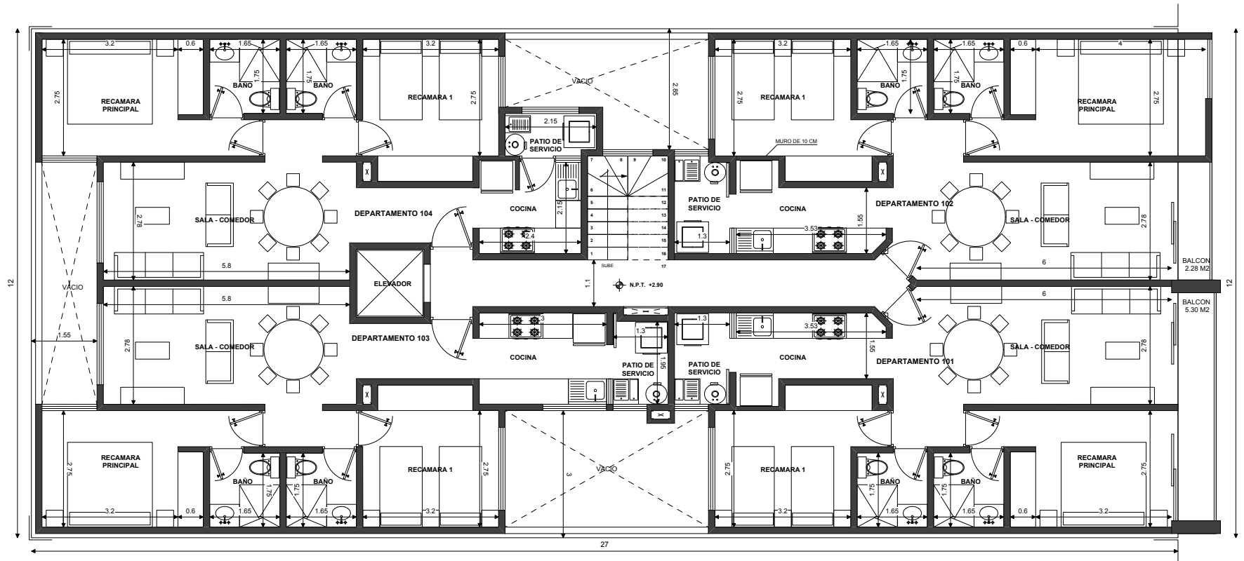
PLANTA N+1
