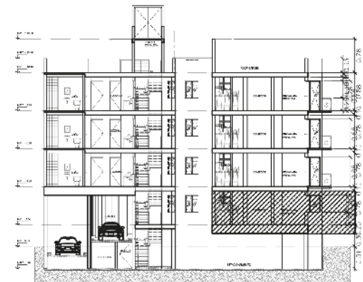
CORTE ESQUEMATICO
