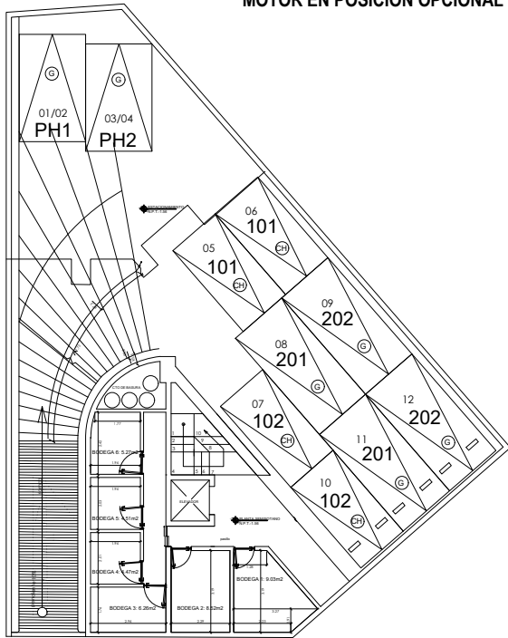
-1 PLANTA SEMISOTANO
