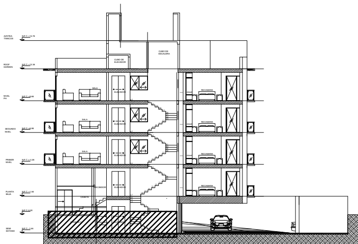
CORTE ESQUEMATICO
