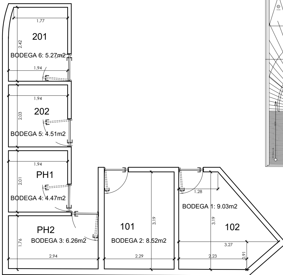
-1 PLANTA SEMISOTANO ARQUITECTONICO
