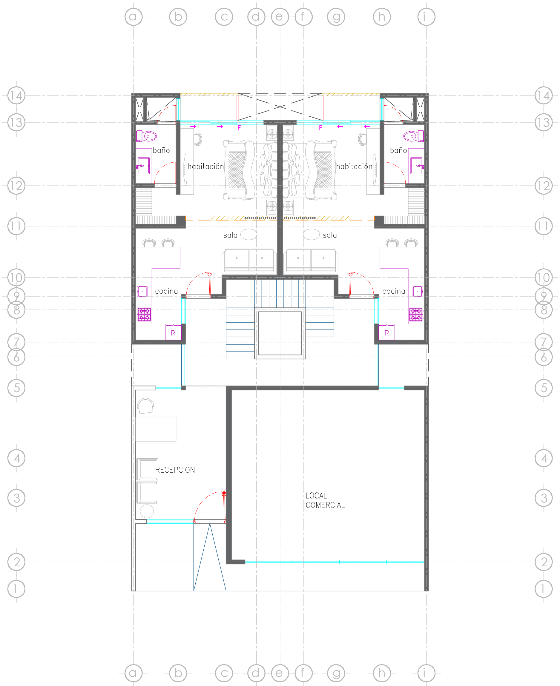
PLANTA BAJA
