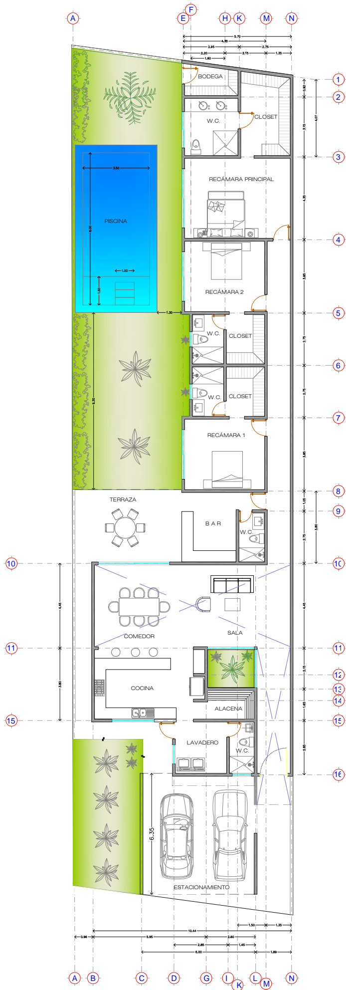
PLANTA ARQUITECTÓNICA MODELO B
