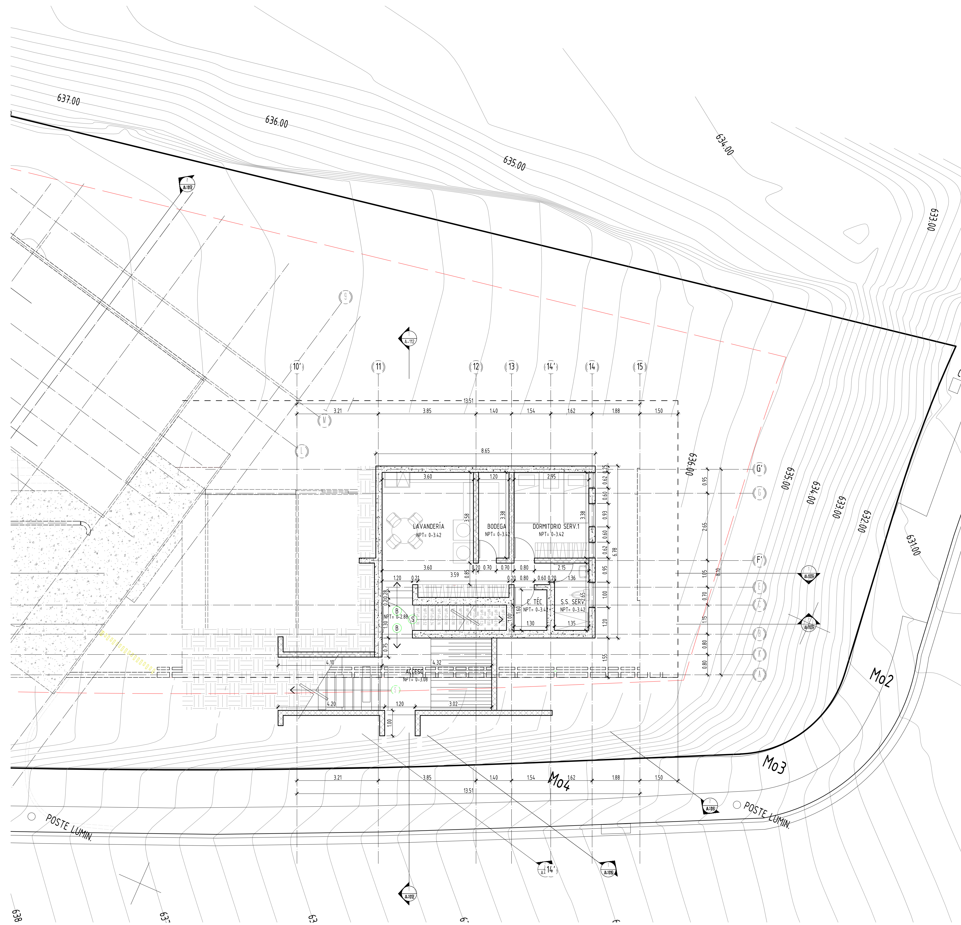
PLANTA ARQUITECTONICA SOTANO 1 1 : 75
