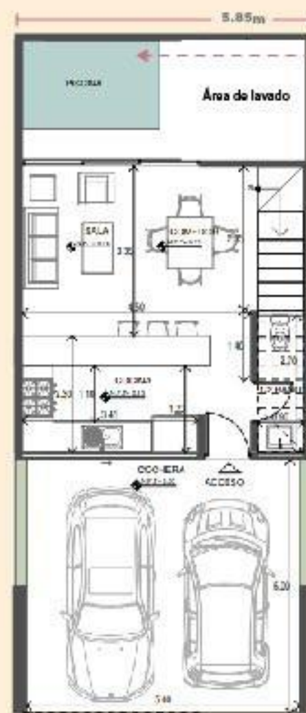
Planta baja
