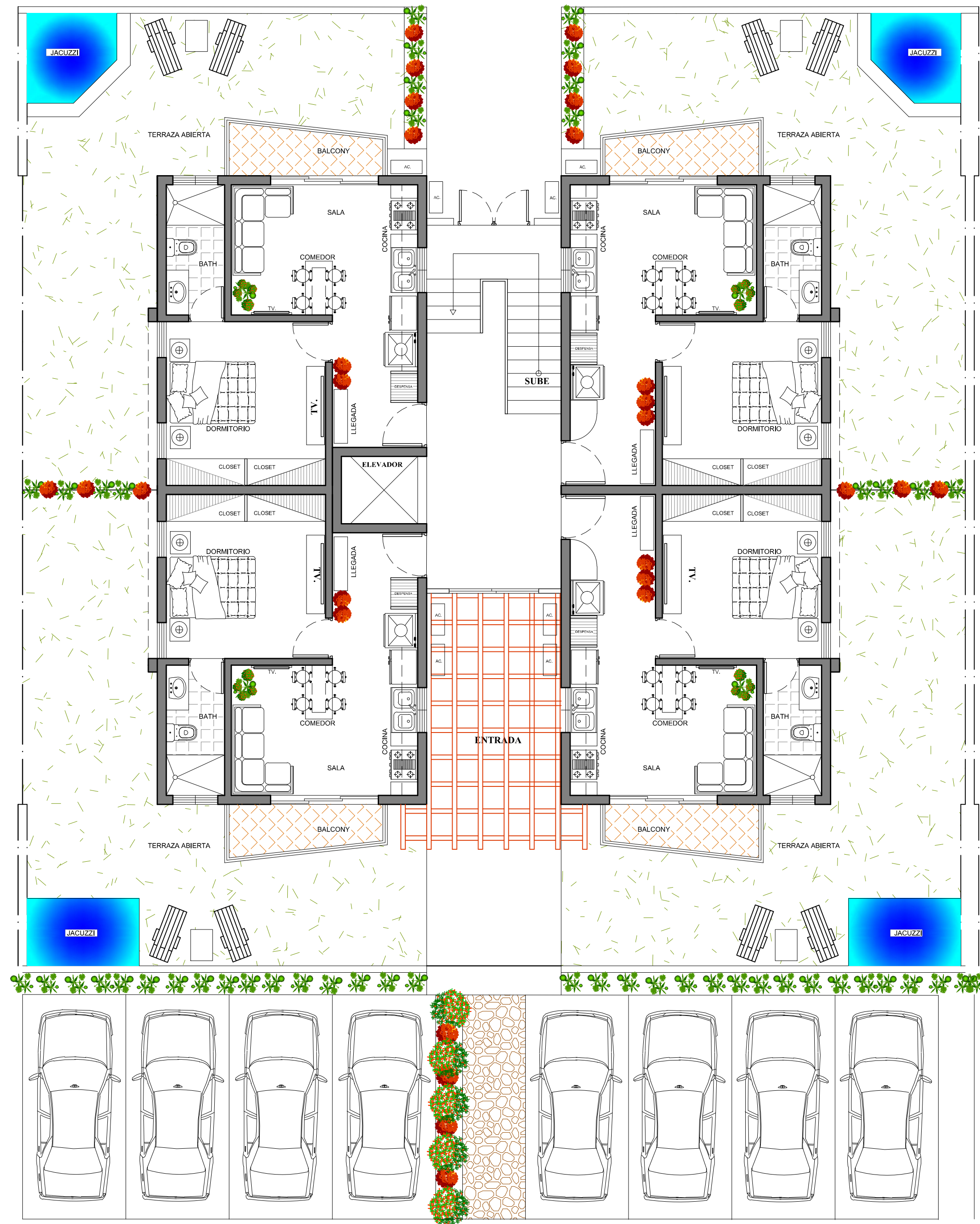
GOLD REEF CITY PLANTA ARQUITECTONICA AMUEBLADA 1ER NIVEL
