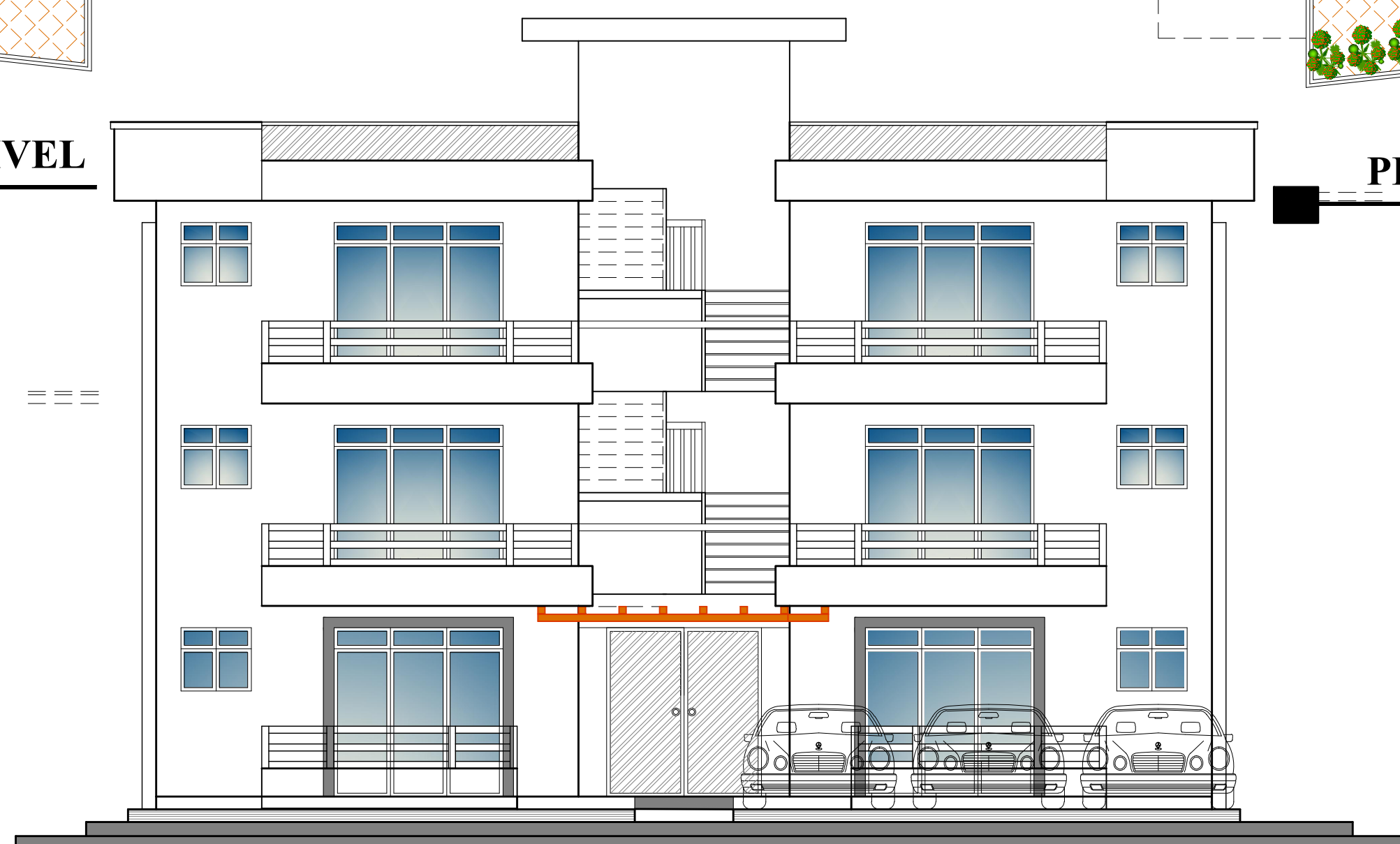
ELEVACION FRONTAL
