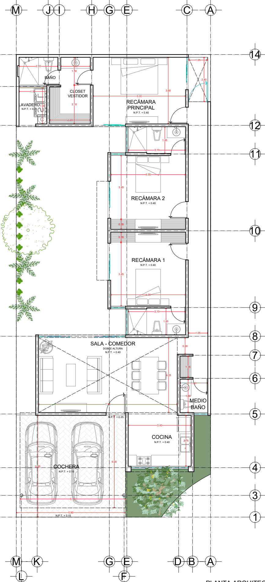
PLANTA ARQUITECTÓNICA
