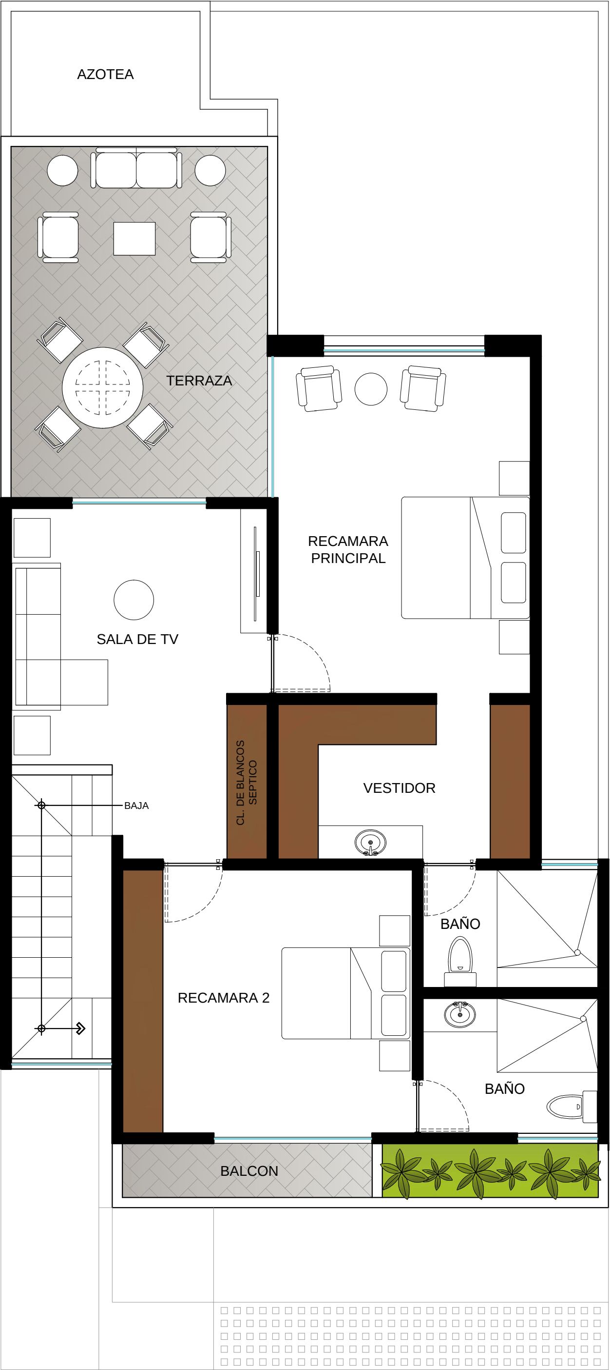
PLANTA ALTA
