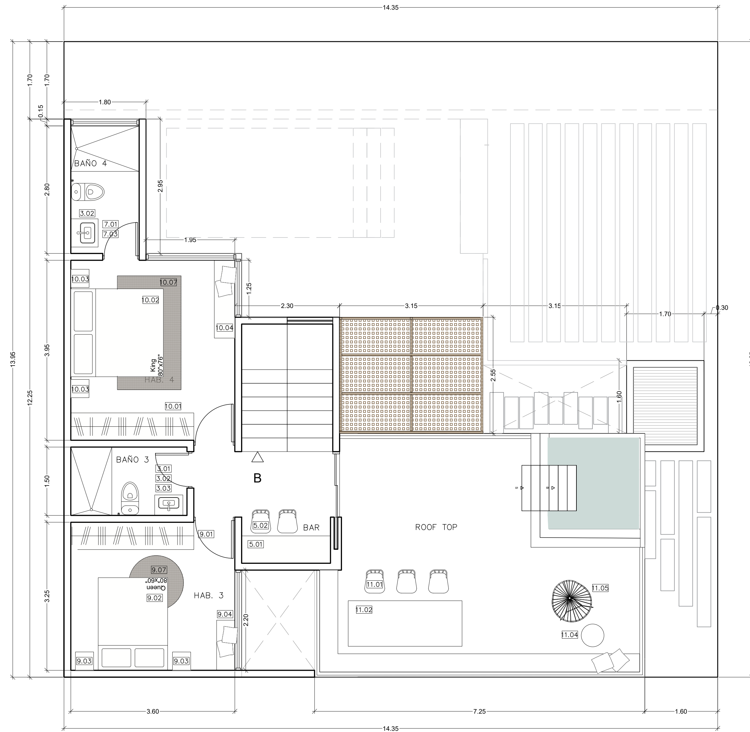
PLANTA DISTRIBUCIÓN DE MOBILIARIO ESC 1:50
