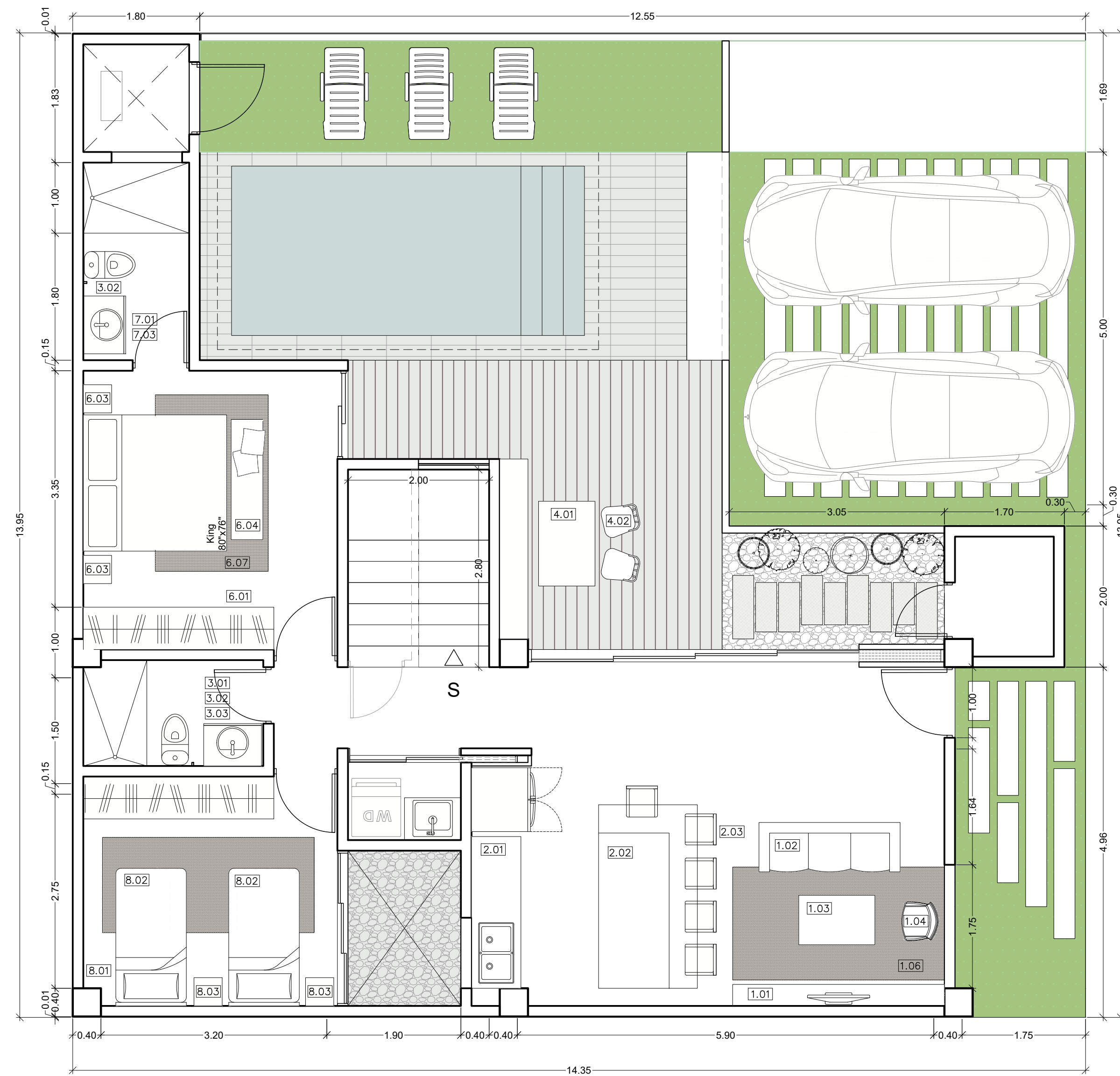
PLANTA DISTRIBUCIÓN DE MOBILIARIO ESC 1:50
