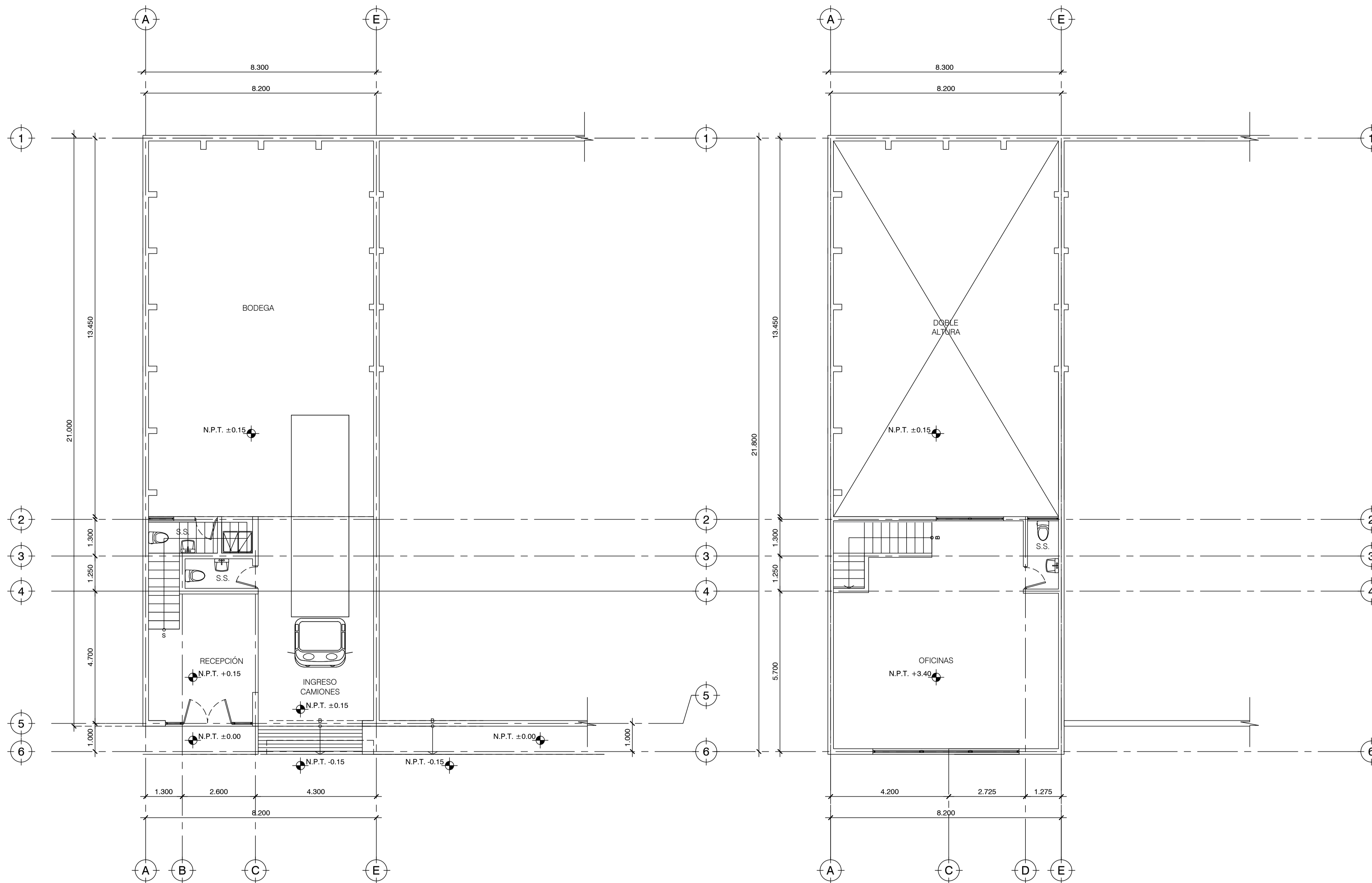
1 PLANTA AMUEBLADA DE OFI-ESPACIO - NIVEL 1 CENTRO DE COMERCIO SANTA FE ESCALA 1 : 75
