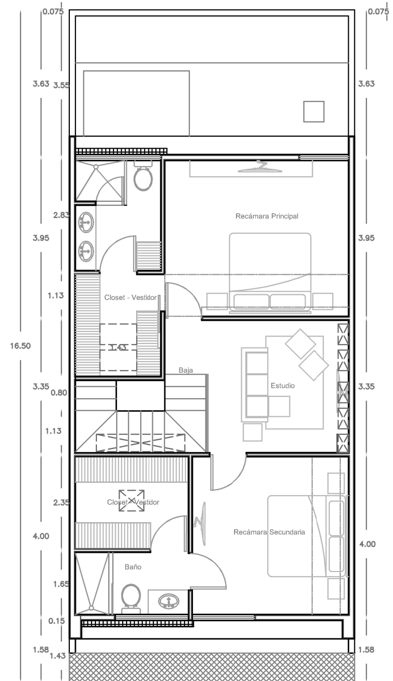
PLANTA ALTA
