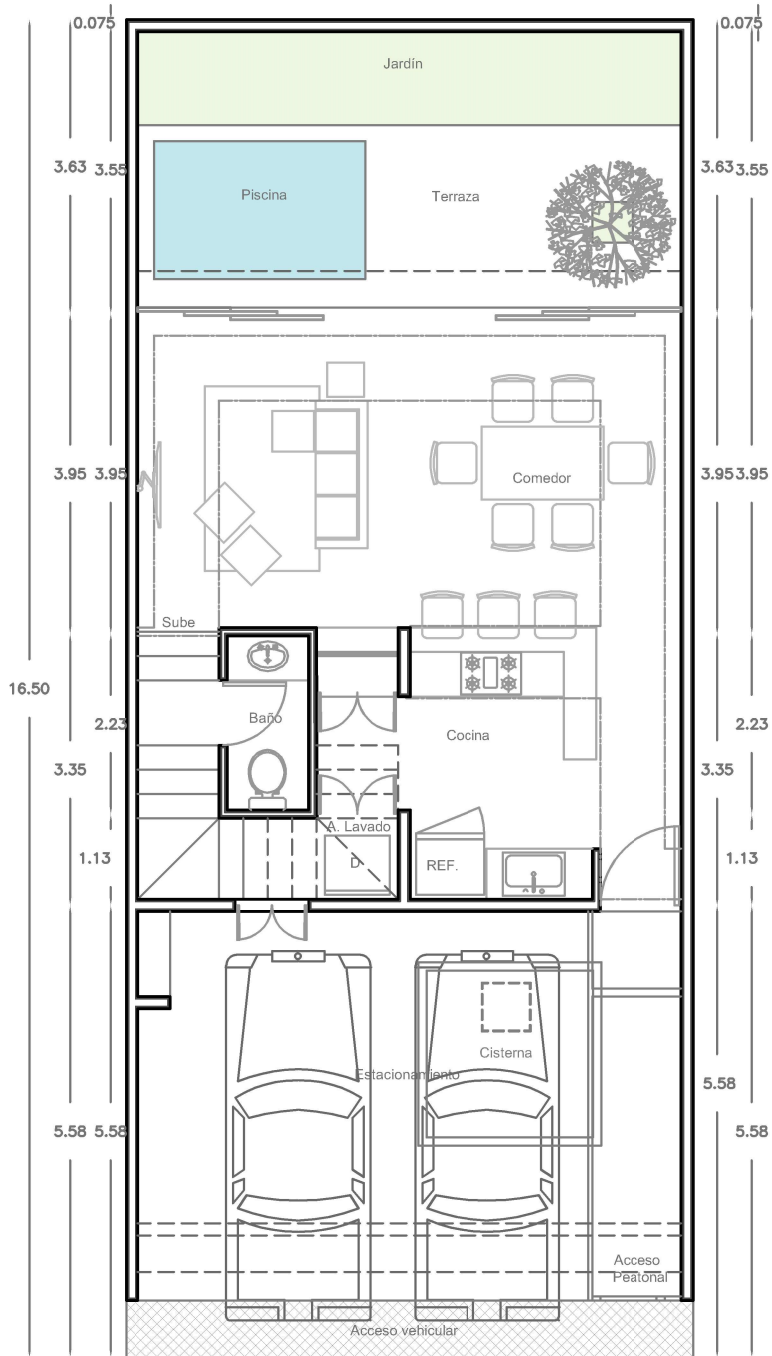
PLANTA BAJA
